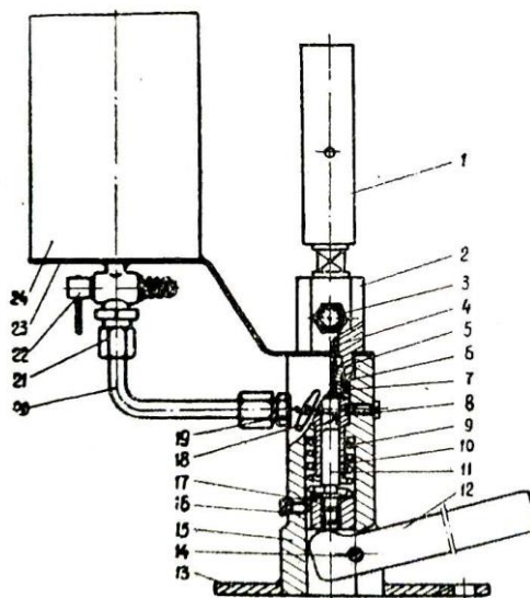
Рисунок 5.1 Прилад для регулювання форсунок.
