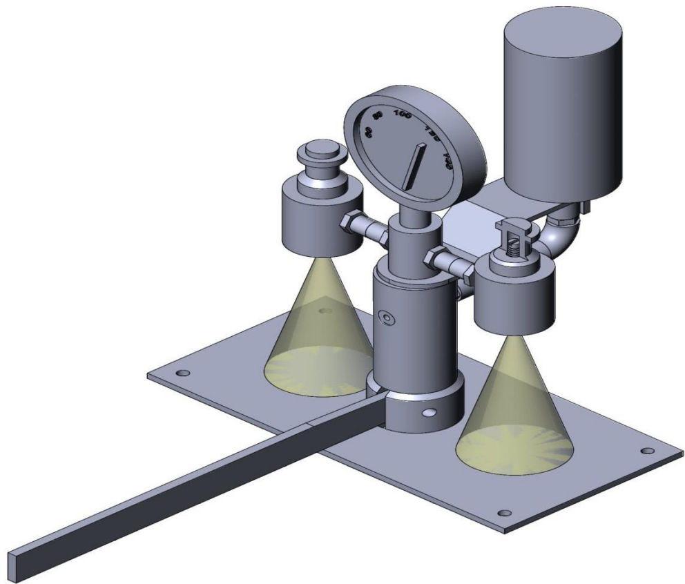
Рисунок 5.2 Схема роботи модернізованого приладу для регулювання форсунок
