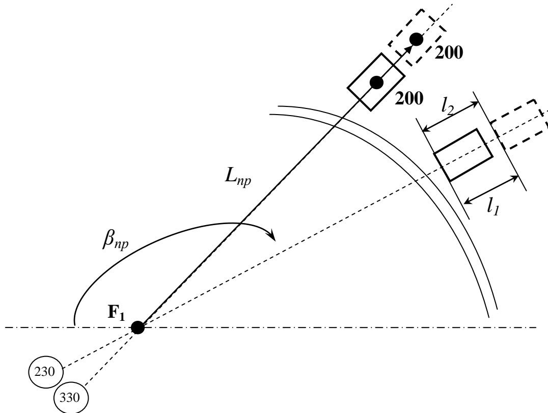
Рис. 6.8. Розмічування еліптичної кривої з точки фокуса
