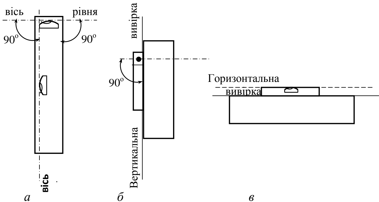
Рис. 7.13. Будівельні рівні
