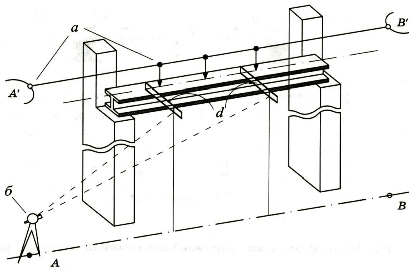
Рис. 8.40. Розмічування для монтажу підкранових рейок:
