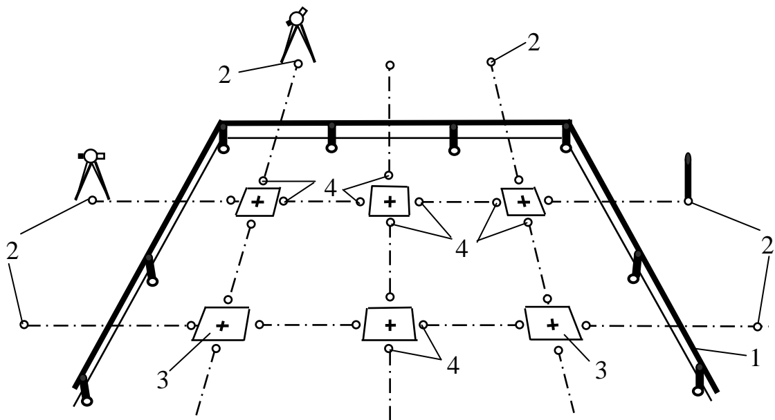
Рис. 8.17. Розмічування осей фундаментів під колони:
