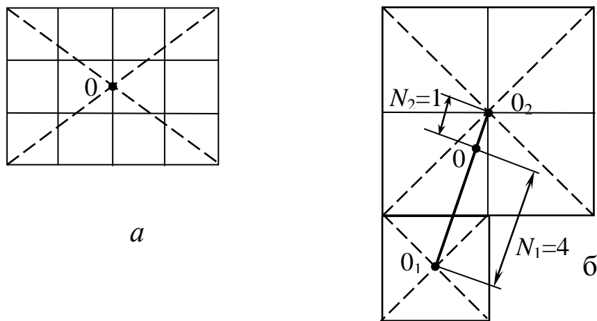
Рис. 4.19. Визначення положення центра ваги
