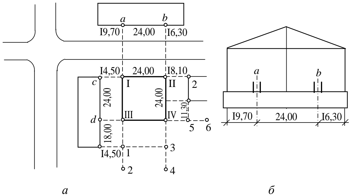
Рис. 8.6. Схема прив'язки осей будинку до місцевих предметів та контурів:
