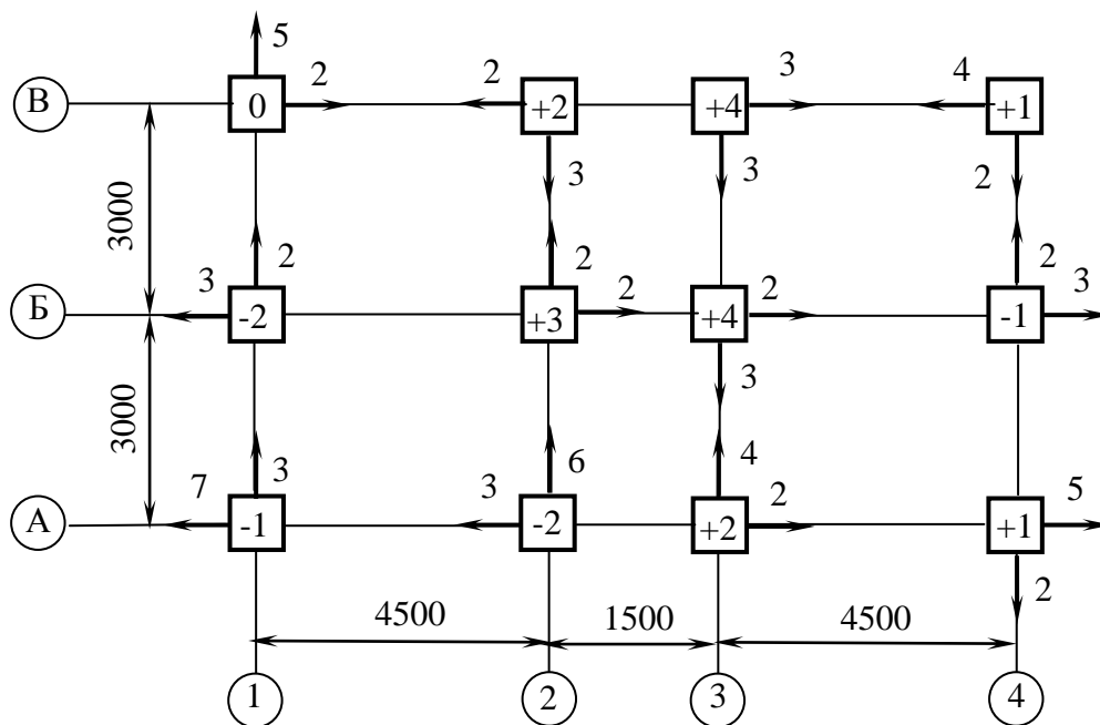
Рис. 8.50. Виконавча схема пальового поля
