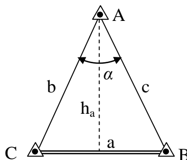
Рис. 2.6. Схема трикутника трилатерації
