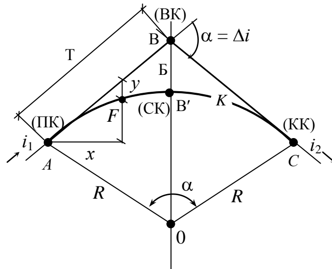
Рис. 6.2. Елементи вертикальної кривої
