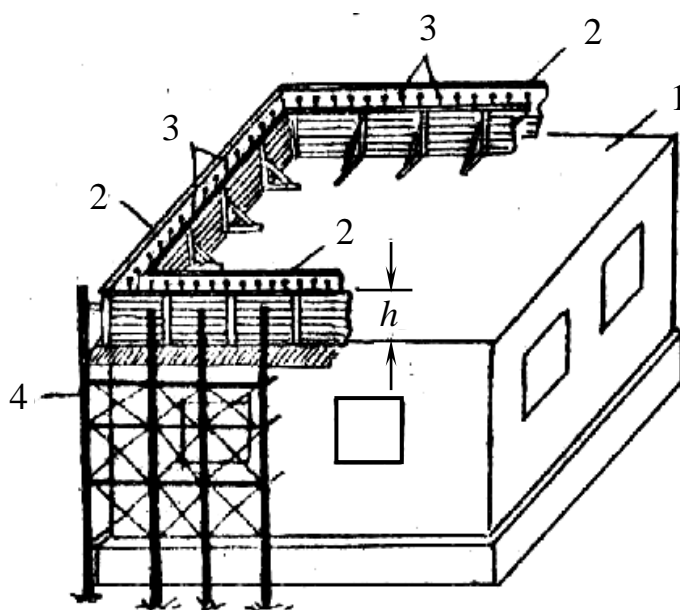
Рис. 8.33. Схема встановлення переставної опалубки:
