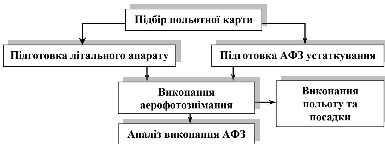
Рис. 3.3. Технологічна схема АФЗ з використанням БПЛА
