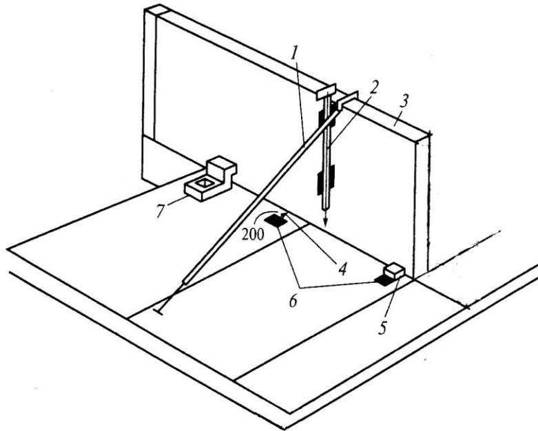
Рис. 8.28. Вивірення панелей:
