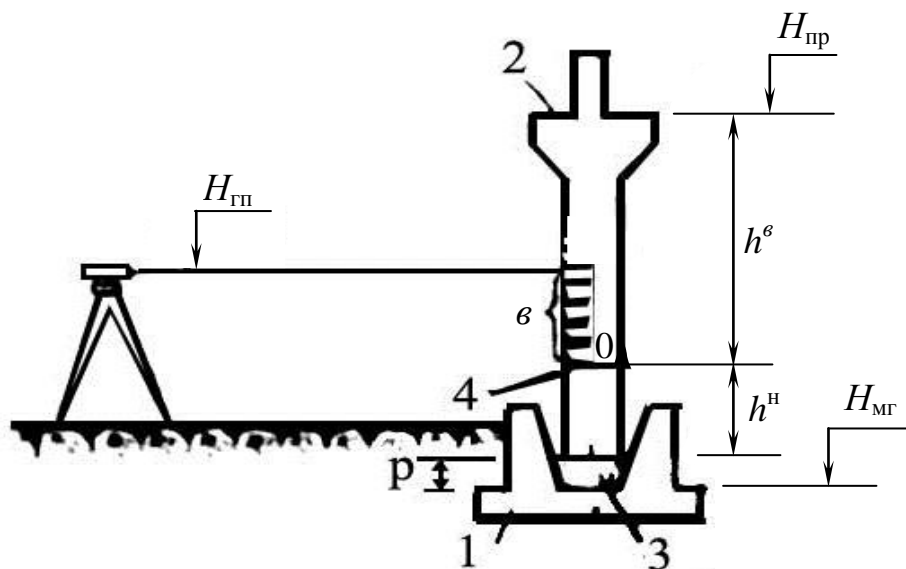
Рис. 7.11 Монтаж збірної залізобетонної колони за висотою
