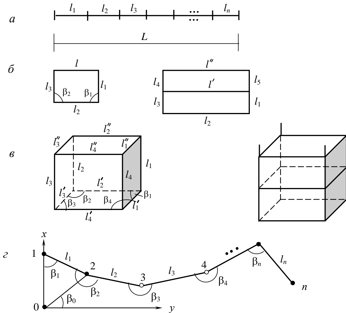
Рис. 4.13. Види розмірних ланцюгів
