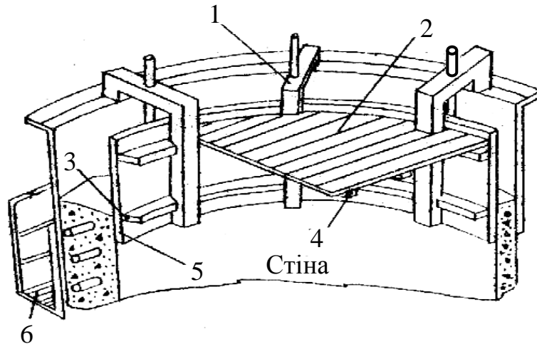
Рис. 8.34. Схема побудови ковзної опалубки:
