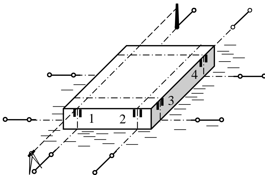
Рис. 8.20. Схема перенесення та закріплення осей на вихідному монтажному горизонті
