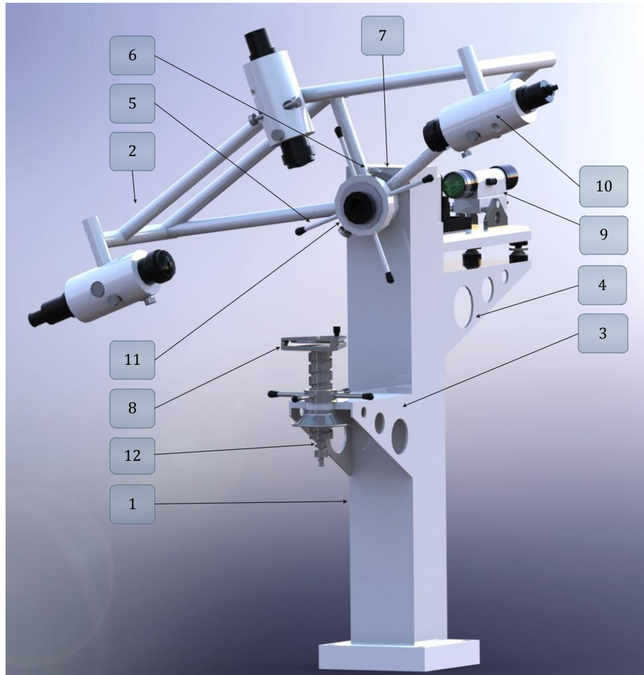
Рис. 10.2. Загальний вигляд автоколімаційної установки для повірки теодолітів і нівелірів АУПНТ
