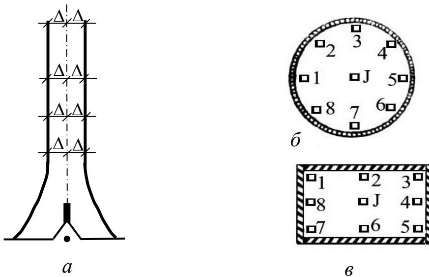
Рис. 7.17. Визначення відхилень способом оптичної вертикалі
