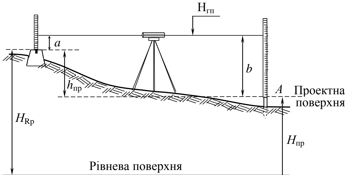
Рис. 5.2. Схема винесення точки із заданою позначкою
