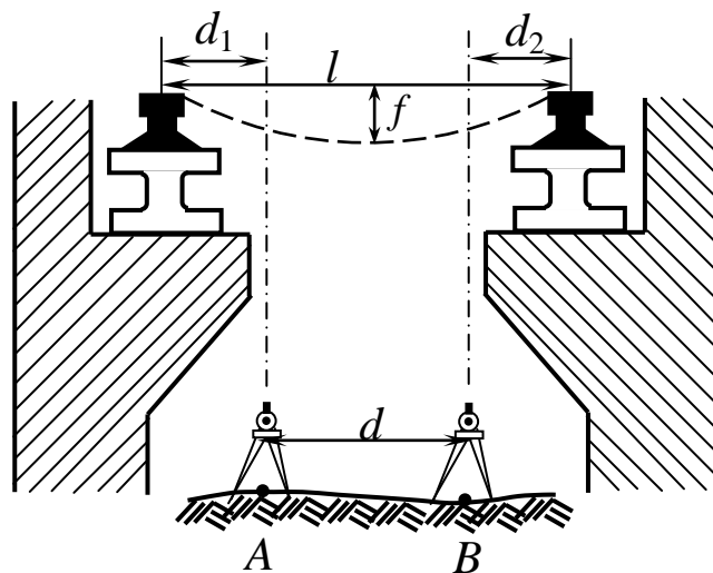
Рис. 8.41. Визначення відстаней між осями підкранових рейок
