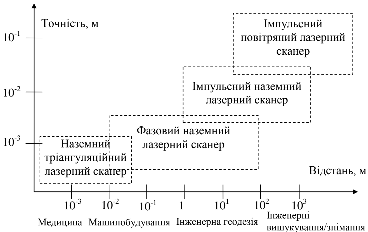
Рис. 3.6 Класифікація систем лазерного сканування
