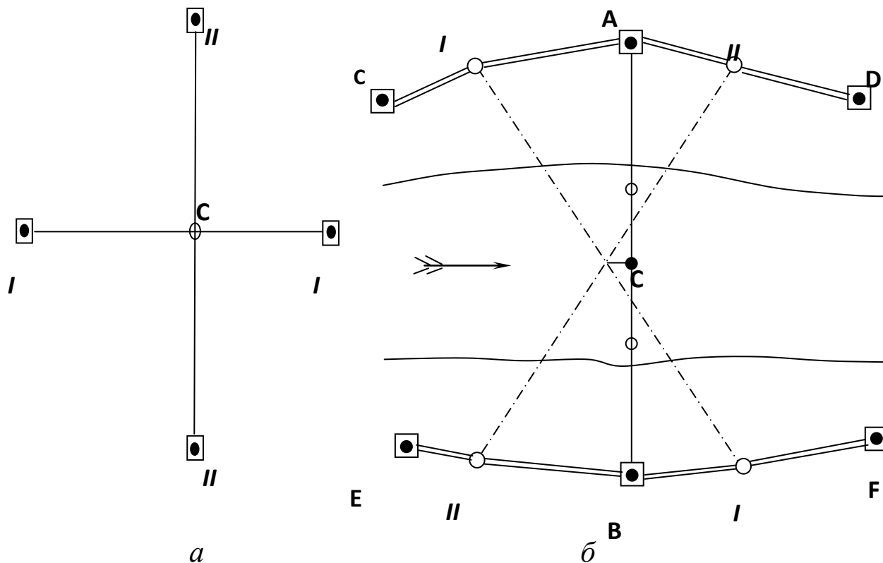
Рис. 5.7. Спосіб створної засічки:
