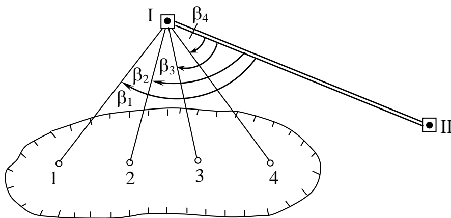
Рис. 9.12. Визначення зсуву методом окремих напрямків
