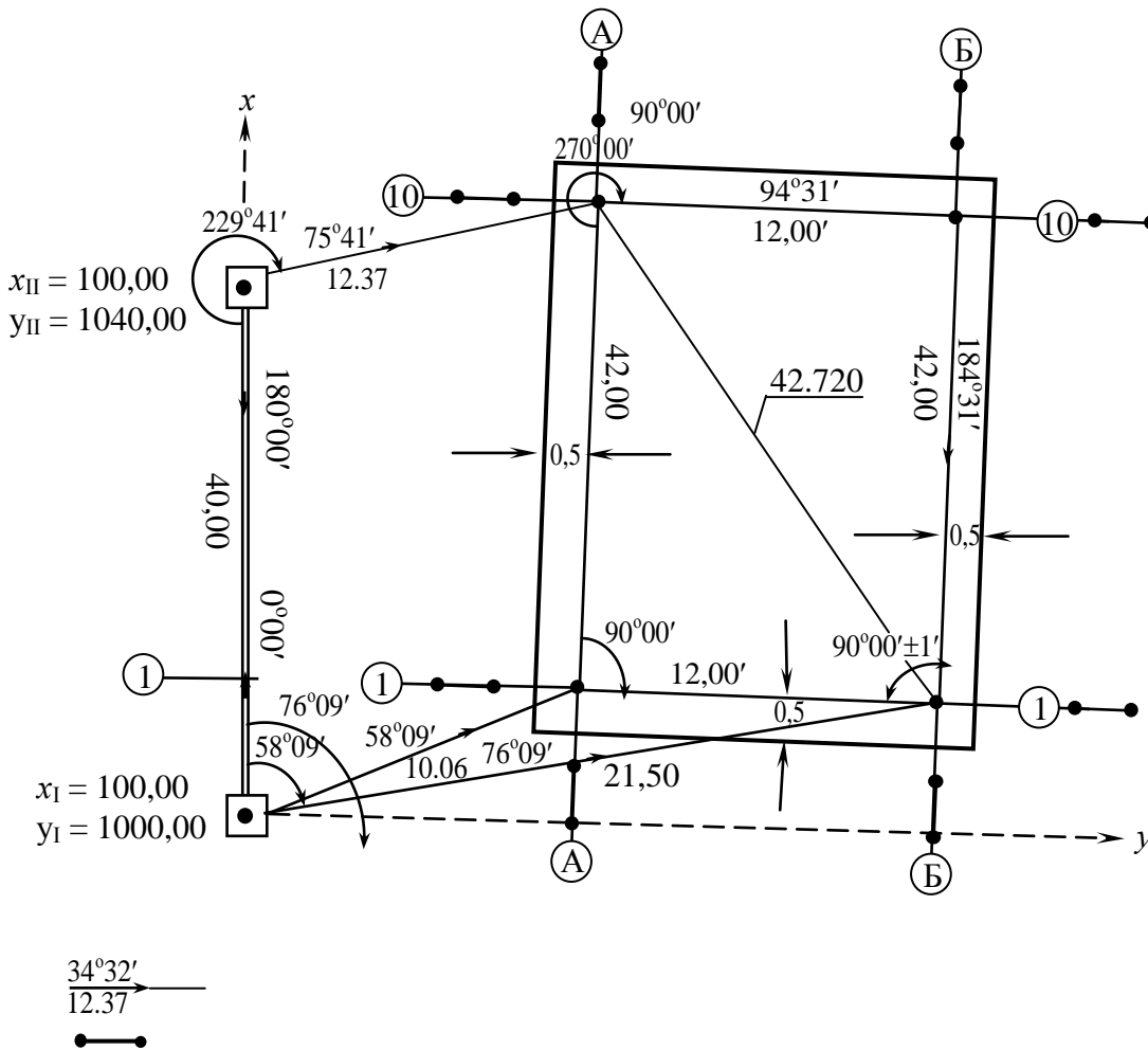
Рис. 4.17. Розмічування основних осей будинку
