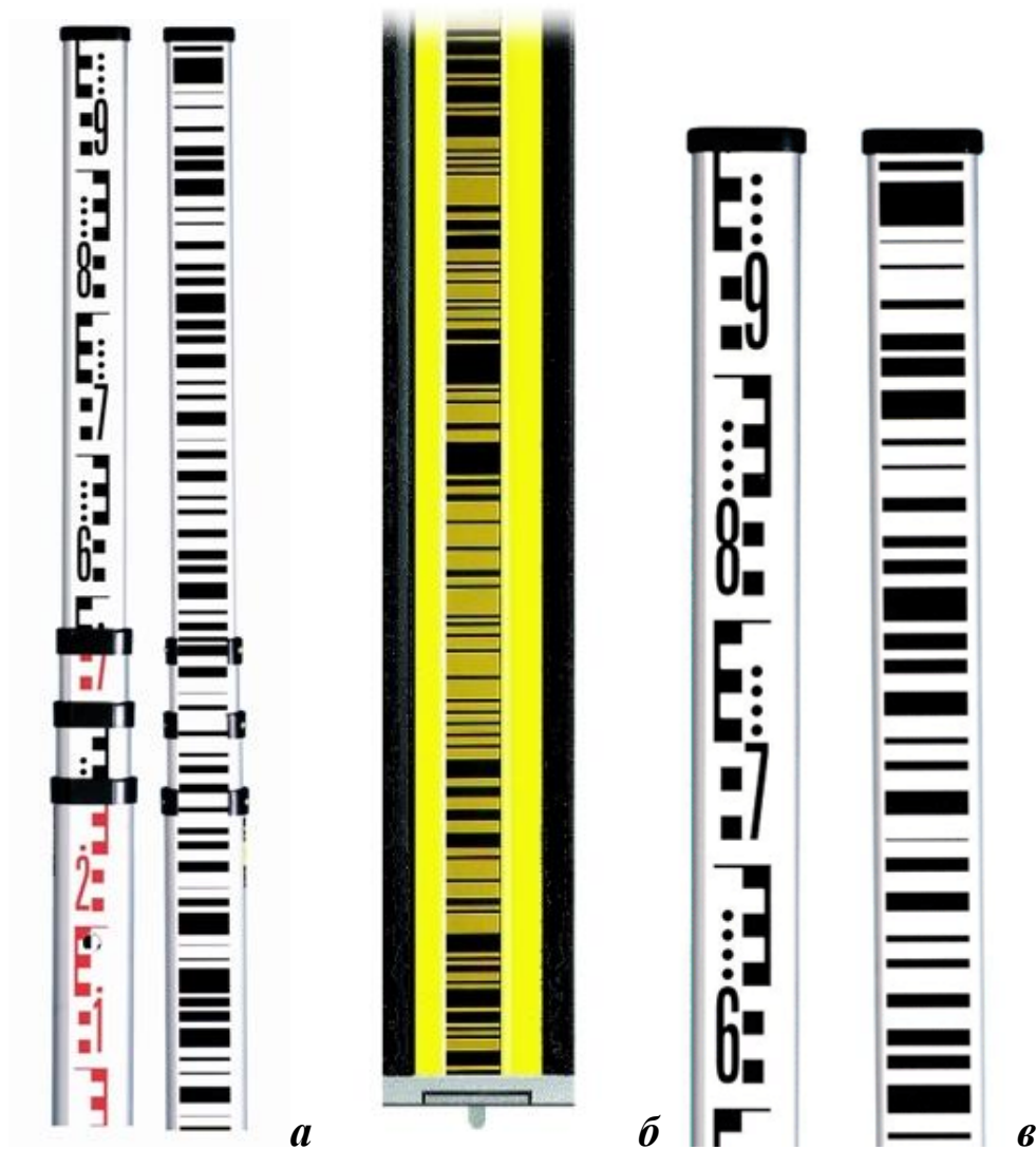
Рис. 1.14. Рейки для цифрових нівелірів
