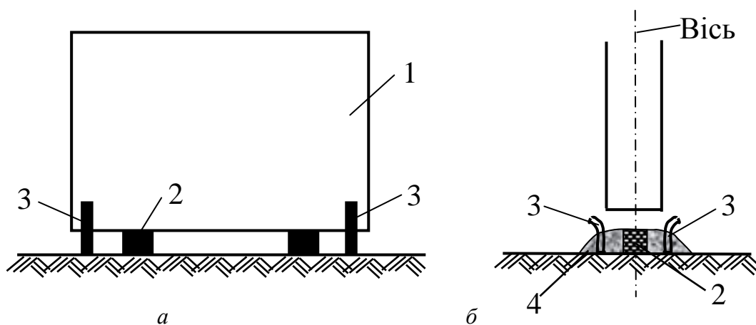
Рис. 8.27. Схема фіксованого монтажу панелей:
