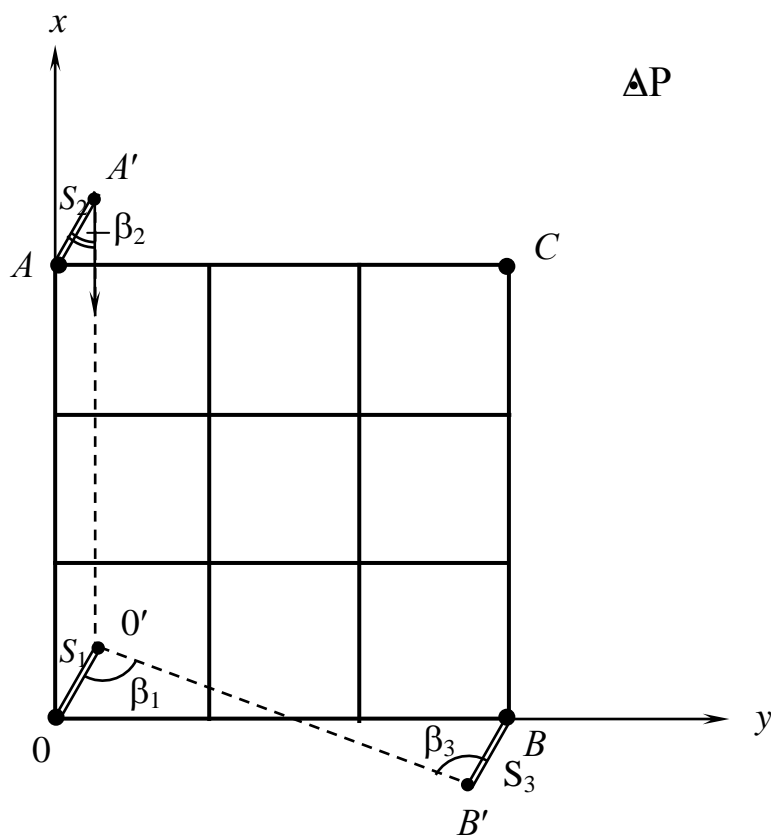
Рис. 4.7. Схема розмічення осей будівельної сітки GPS-методом
