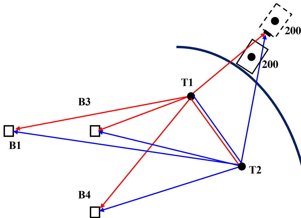
Рис. 6.10. Схема розмічування колової кривої методом вільної станції з контролем
