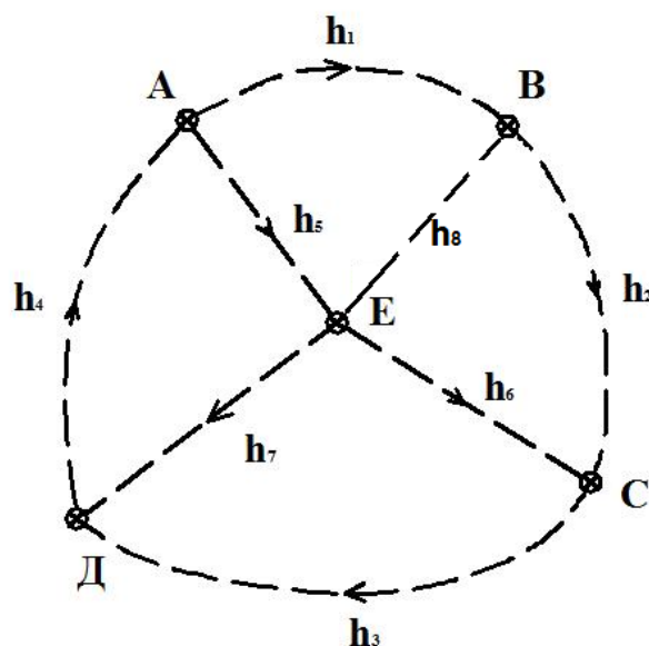
Рис. 2.18. Схема нівелірної мережі
