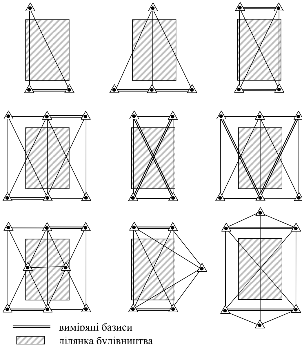
Рис. 2.4. Схеми інженерно-геодезичних мереж триангуляції
