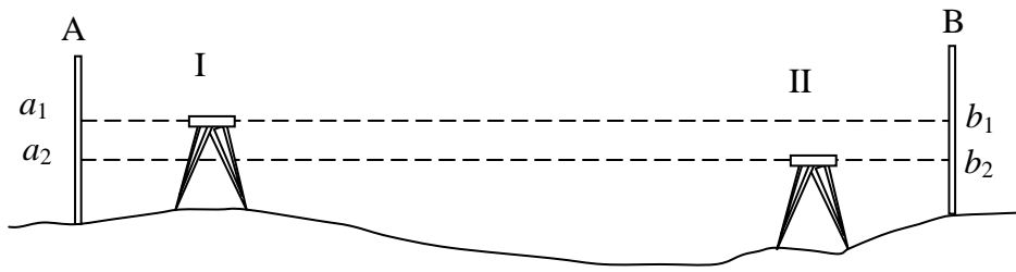
Рис. 10.10. Перевірка кута неузгодженості візирної осі нівеліра
