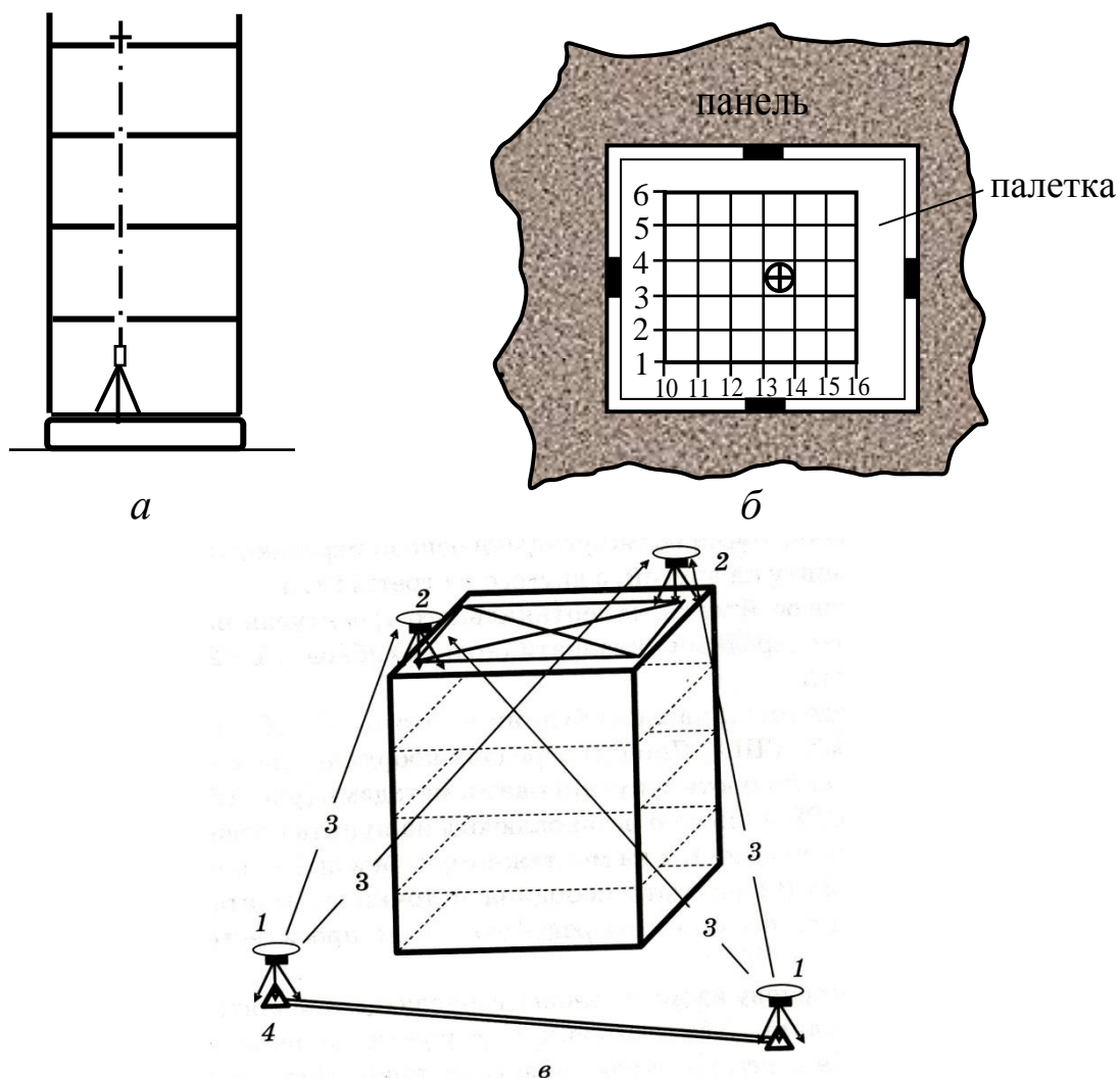
Рис. 8.23. Способи вертикального проектування (а,б) та GPS-спостережень
