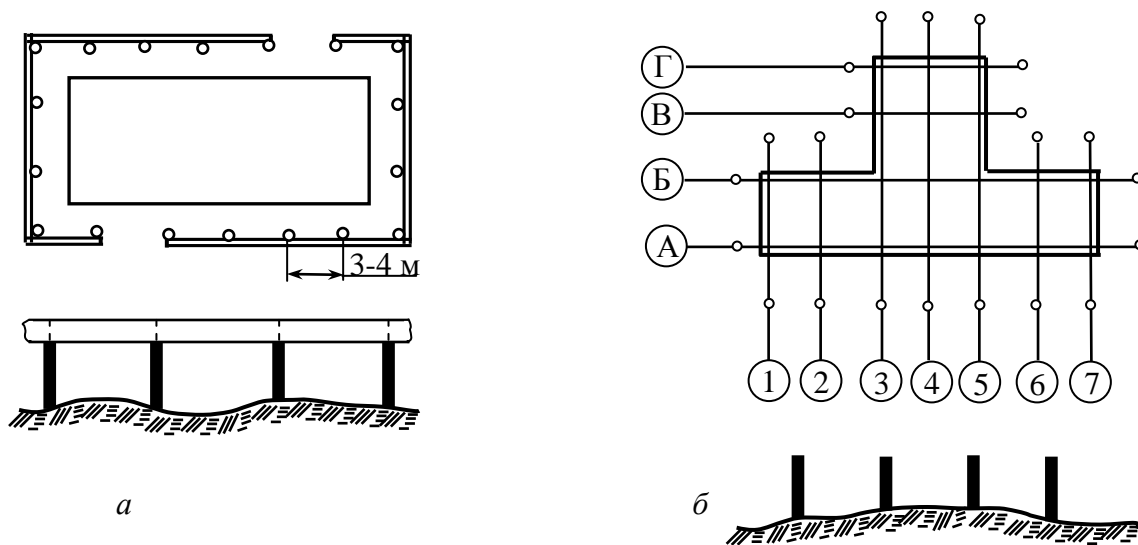
Рис. 8.7. Схема побудови обноски: а – суцільна; б – створна
