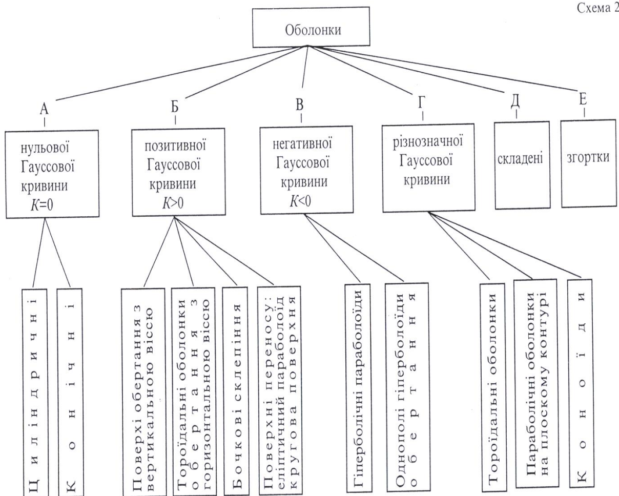
Рис. 6.12. Класифікація просторових оболонок
