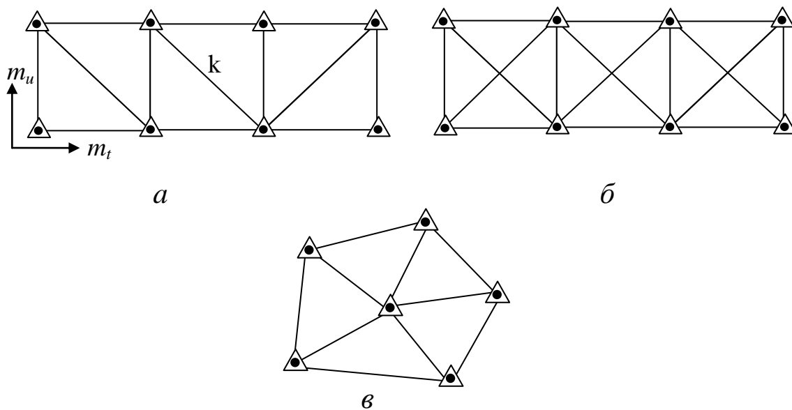
Рис. 2.5. Схеми мереж трилатерації
