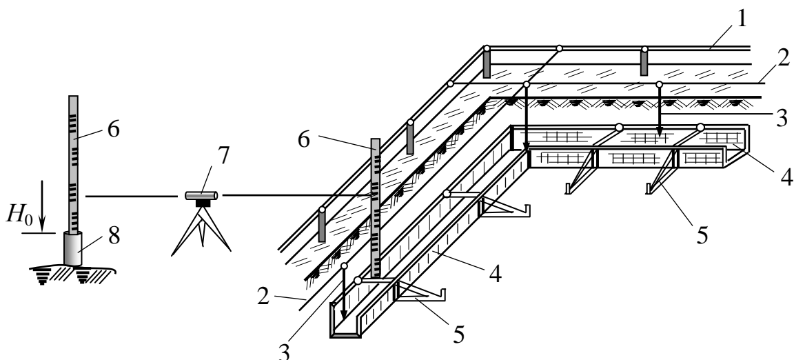
Рис. 8.16. Монтаж опалубки стрічкового фундаменту:
