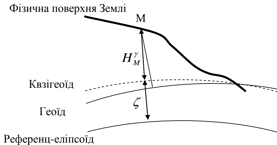
Рис. 2.17. Відлікові поверхні
