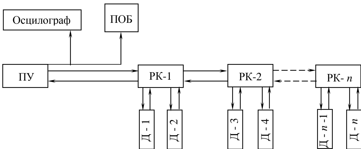
Рис. 9.6. Електрична блок-схема гідростатичної системи
