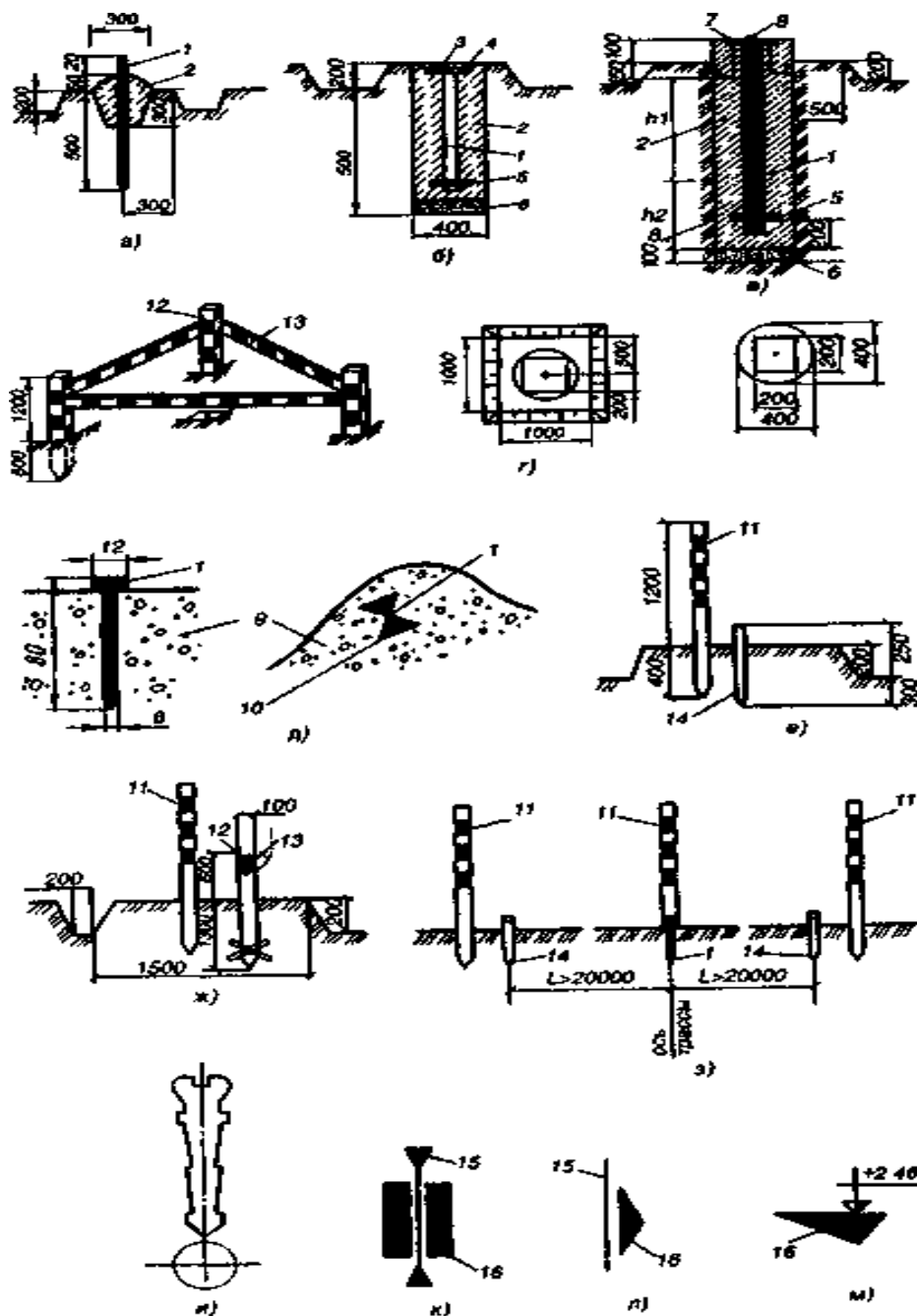
Рис. 2.24. Знаки закріплення інженерно-геодезичних мереж
