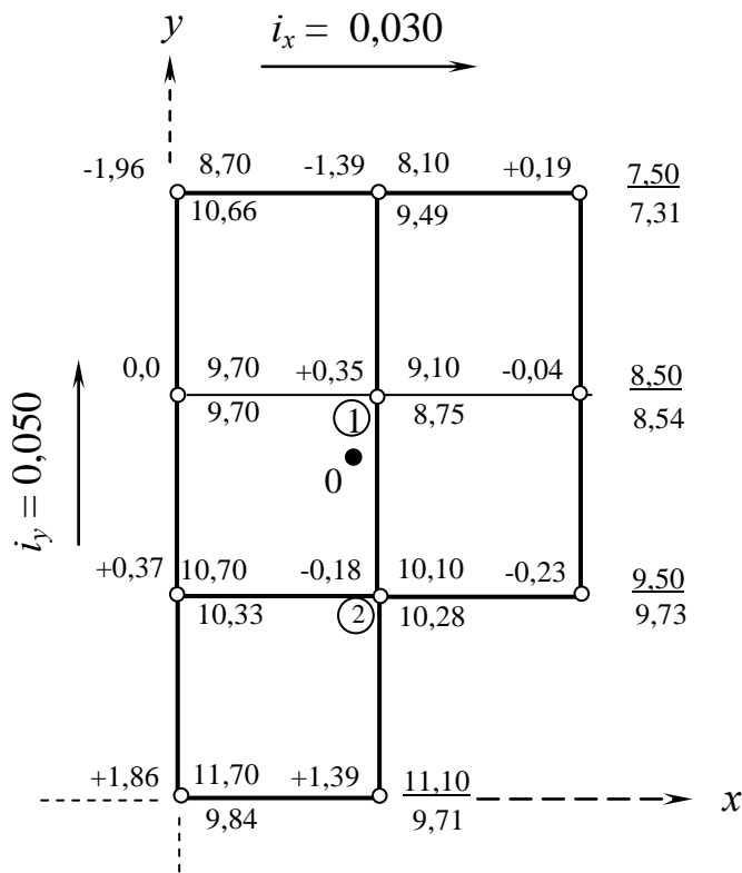
Рис. 4.20. Проектування нахиленої площини
