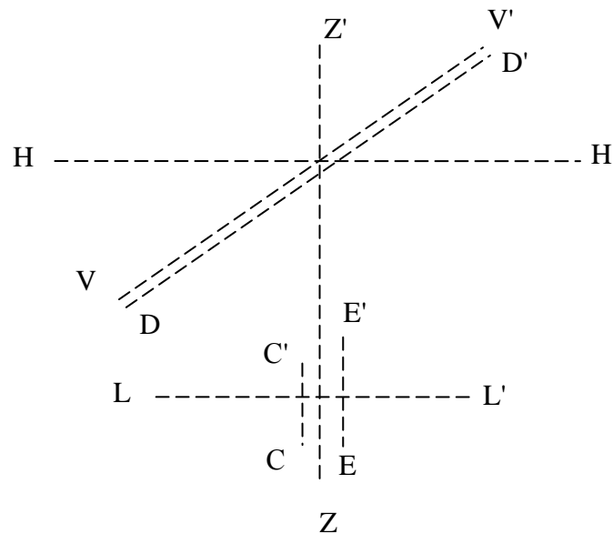
Рис. 10.5. Схема осей електронного тахеометра
