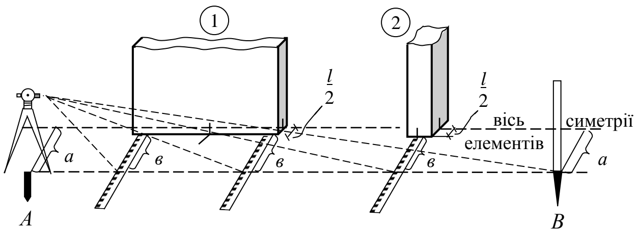
Рис. 7.5. Схема способу бокового нівелювання:
