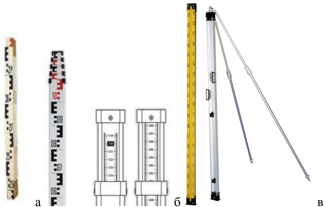
Рис. 1.13. Рейки для оптичних нівелірів
