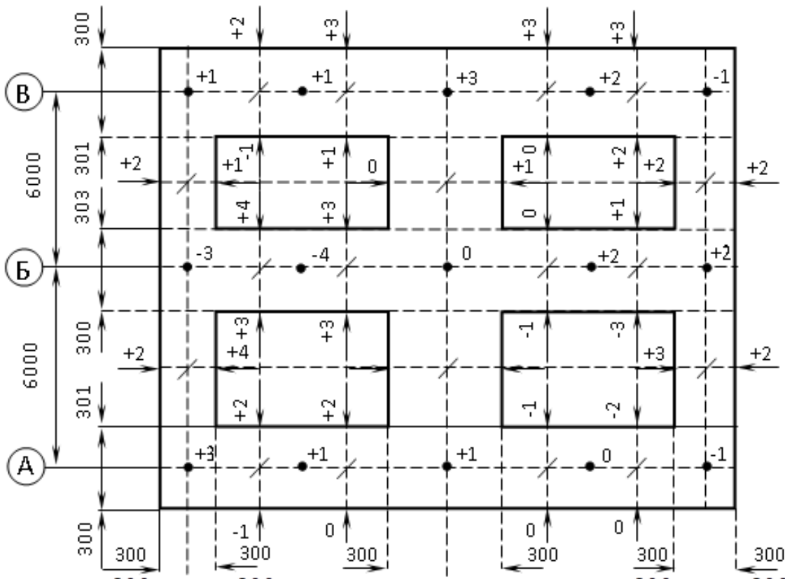
Рис. 8.51. Виконавча схема ростверку
