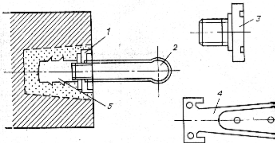
Рис. 9.2. Стінна деформаційна марка
