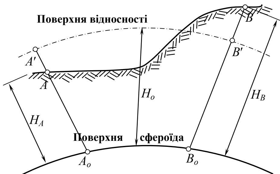
Рис. 4.2. Проектування ліній на поверхню відносності
