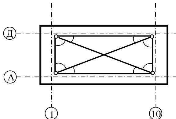
Рис. 8.21. Схема побудови розмічувальної основи
