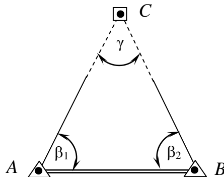
Рис. 2.9. Пряма одноразова кутова засічка
