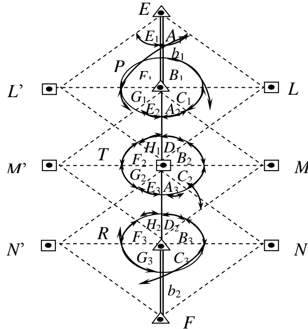
Рис. 2.10. Схема засічки проф. А.І. Дурнева
