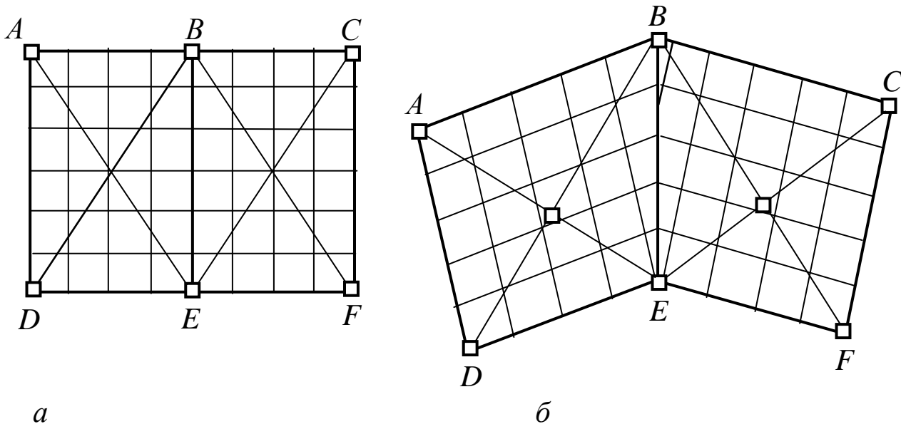
Рис. 4.10. Типи фігур побудови будівельної сітки
