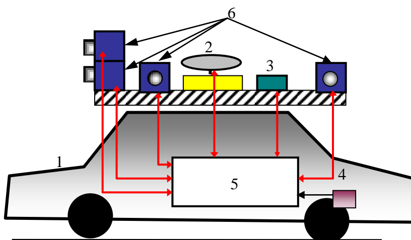
Рис. 3.8. Структурна схема мобільної картографічної системи
