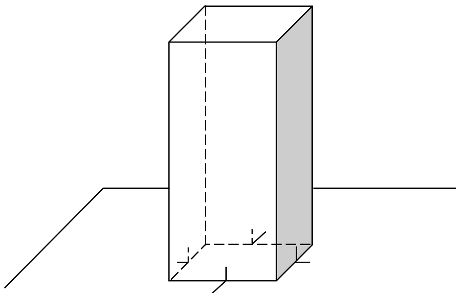
Рис. 7.3. Схема розмічування осей при монтажі колон
