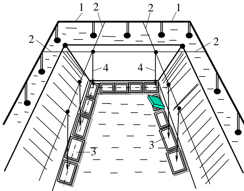
Рис. 8.15. Монтаж блоків стрічкового фундаменту
