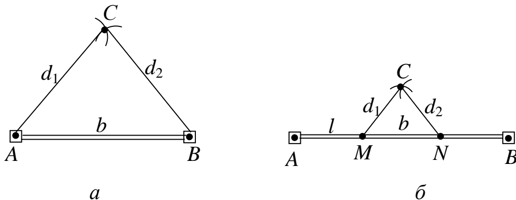
Рис. 5.6. Схема способу лінійної засічки
