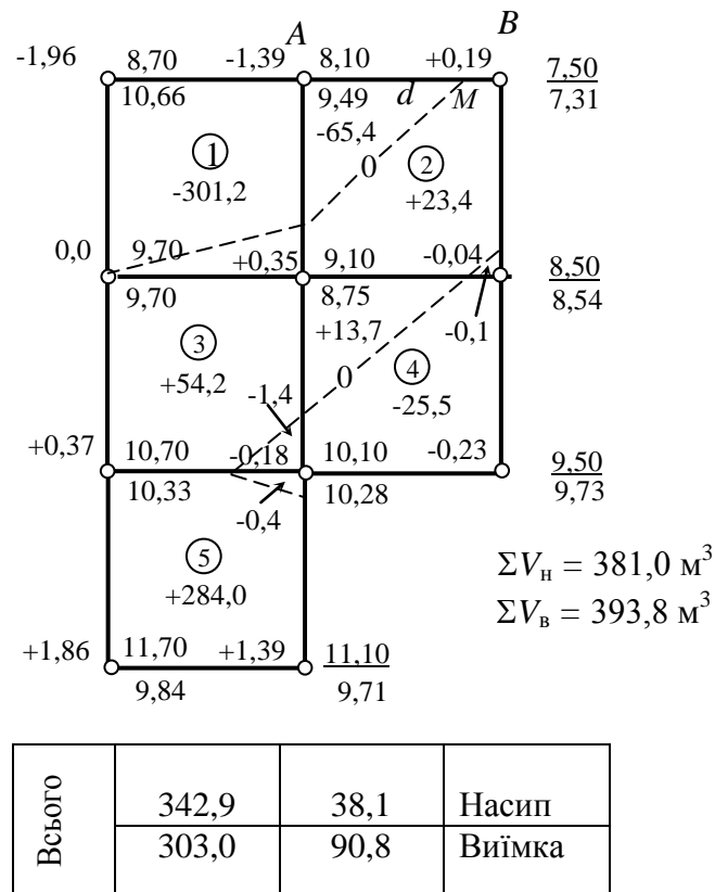
Рис. 4.21. Картограма земляних робіт
