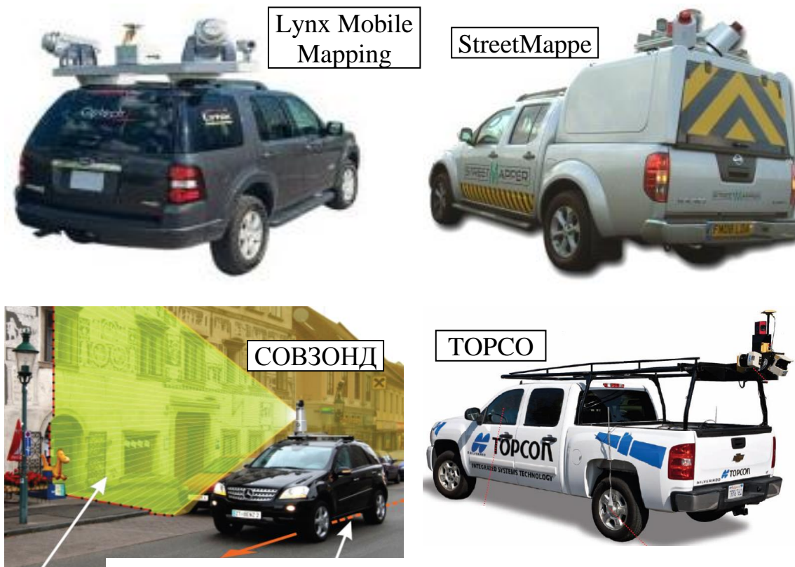
Рис. 3.10. Мобільні лазерні комплекси
