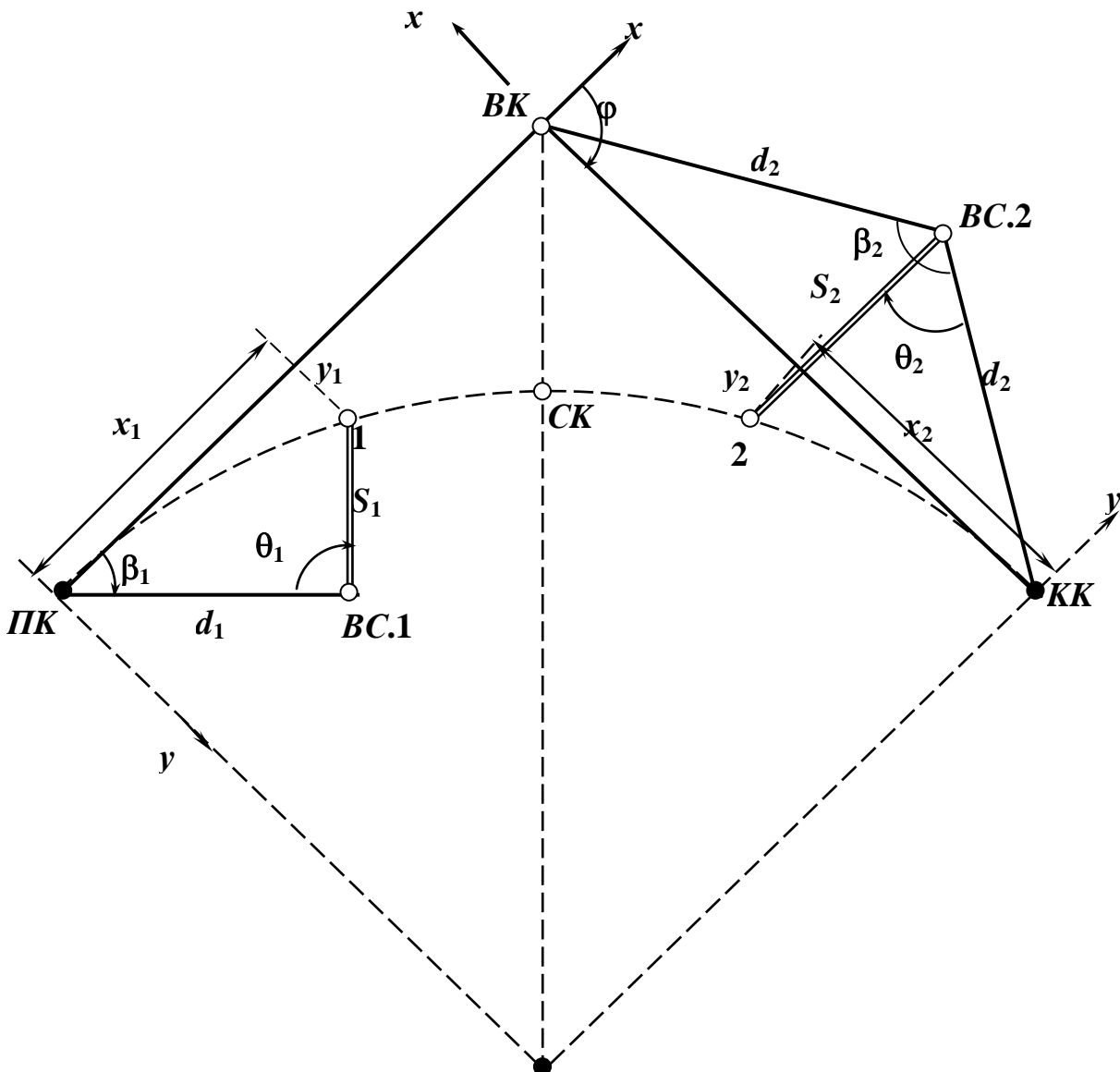
Рис. 6.9. Схема розмічування колової кривої методом вільної станції
