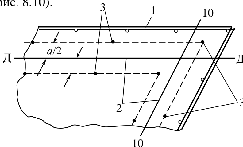
Рис. 8.10. Розмічування котловану під стрічковий фундамент:
