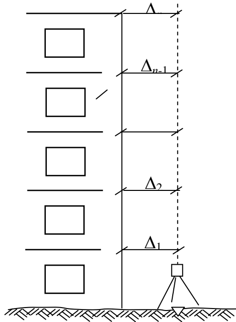
Рис. 9.9. Визначення крену висотного будинку
