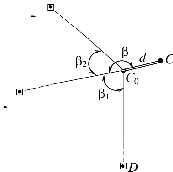
Рис. 5.10. Схема способу оберненої кутової засічки
