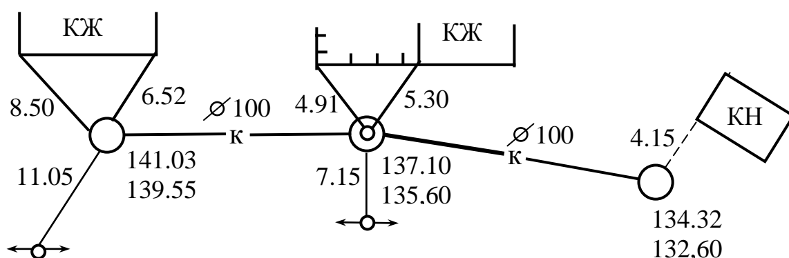
Рис. 8.55. Виконавча схема лінії водопроводу
