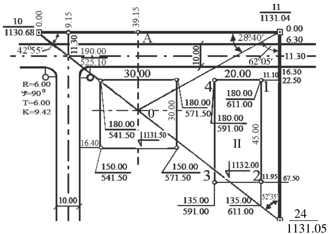
Рис. 4.15. Геодезична підготовка проекту
