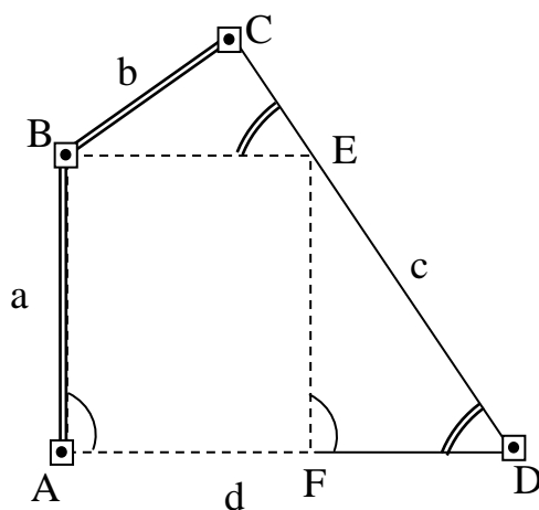
Рис. 2.13. Схема елементарного чотирикутника без діагоналей
