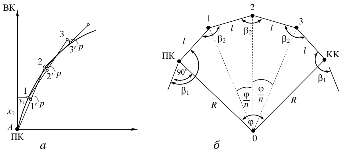
Рис. 6.6. Спосіб трьох точок (а) та вписаного багатокутника (б)
