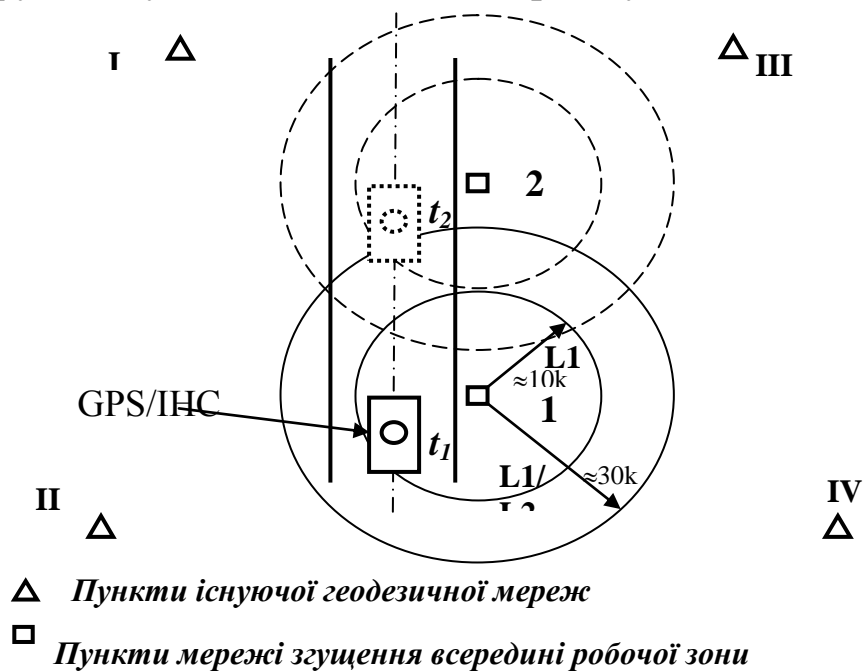
Рис. 3.9. Кінематичне GNSS-знімання лінійного об'єкту
