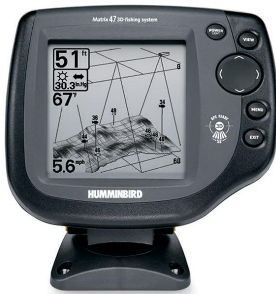
Рис. 3.17. Результати знімання на дисплеї ехолота
