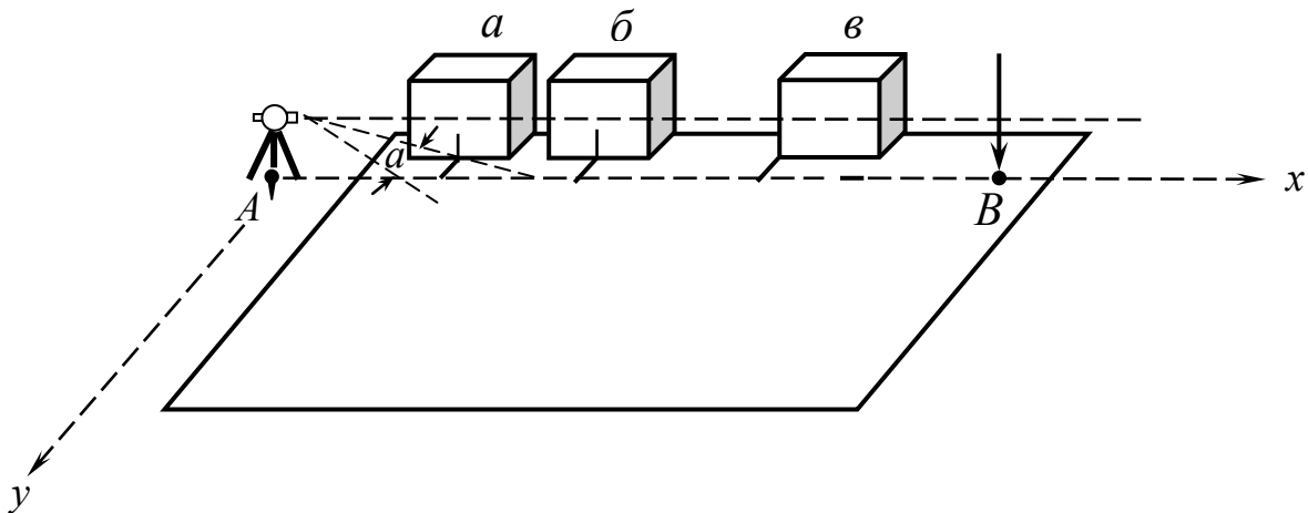
Рис. 7.2. Схема детального розмічування осей при монтажі стінових панелей
