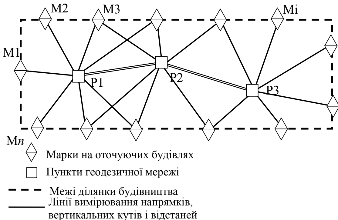
Рис. 2.23. Згущення просторової геодезичної мережі методом вільної станції
