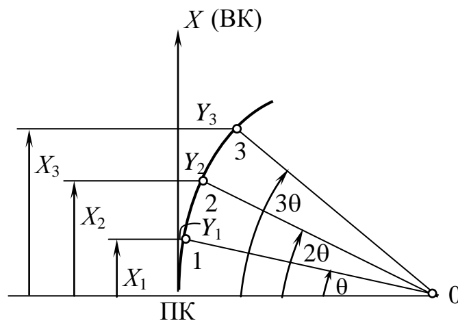
Рис. 6.3. Спосіб прямокутних координат
