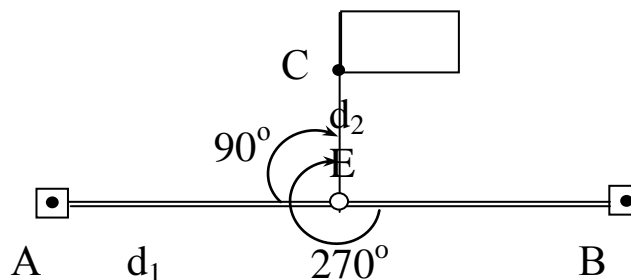
Рис. 5.3. Спосіб прямокутних координат
