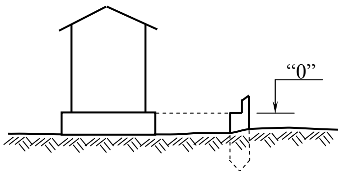
Рис. 4.5. Схема закріплення будівельного нуля
