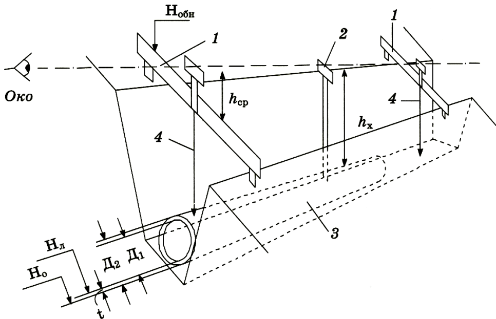
Рис. 8.42. Укладання труб за допомогою візирок: 1 – постійна візирка; 2 – ходова візирка; 3 – труба; 4 – висок
