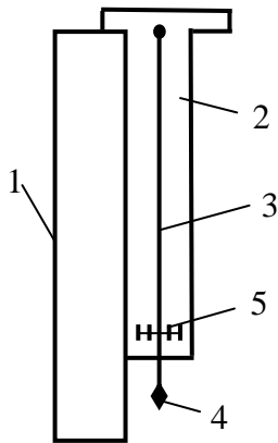
Рис. 7.14. Висок-рейка
