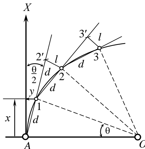
Рис. 6.5. Спосіб продовжених хорд
