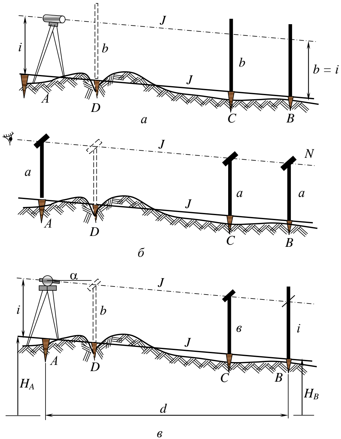
Рис. 5.13. Розмічування лінії заданого нахилу: a – за допомогою нівеліра; б – із застосуванням візирок; в – за допомогою теодоліта
