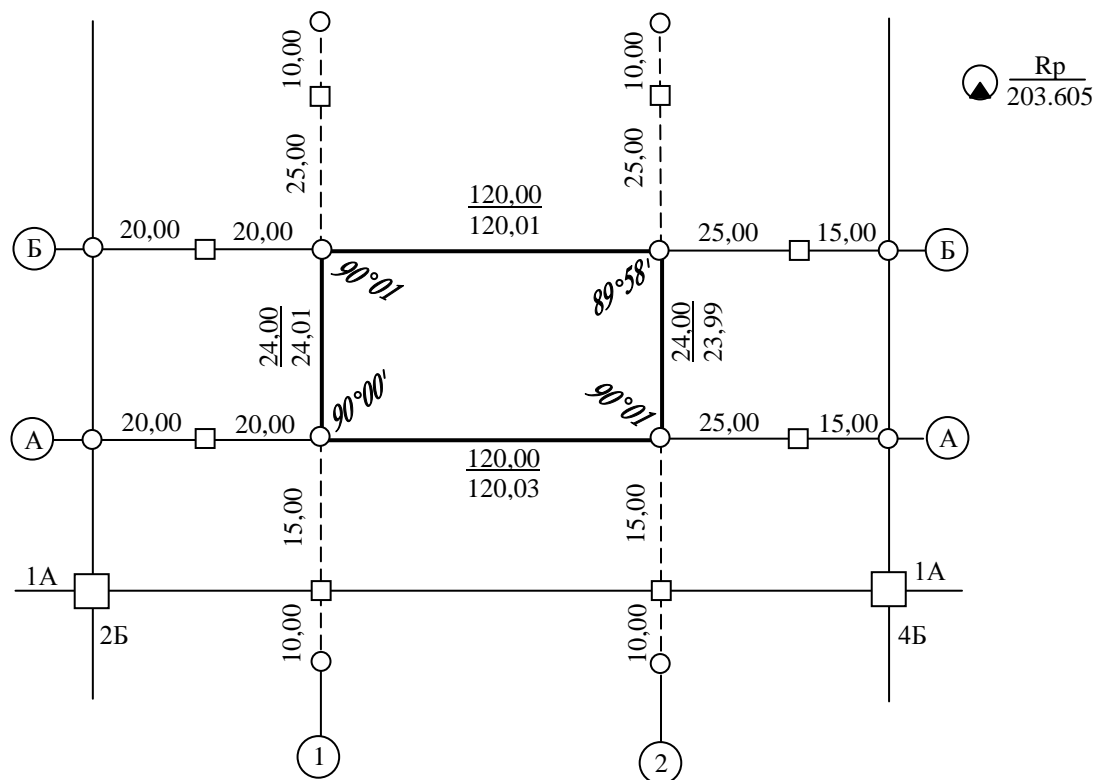
Рис. 8.47. Виконавча схема розмічування і закріплення осей
