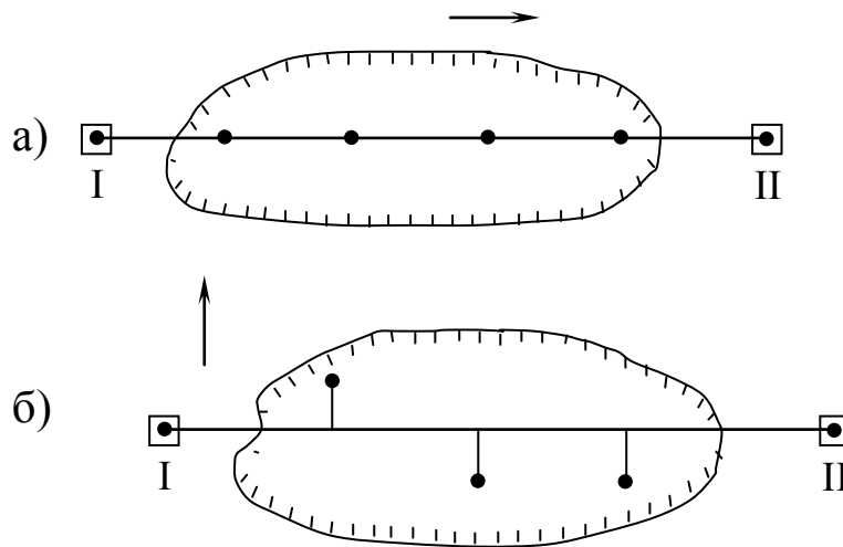
Рис. 9.11. Схема вимірювання зсувів a – метод відстаней; б – метод створів
