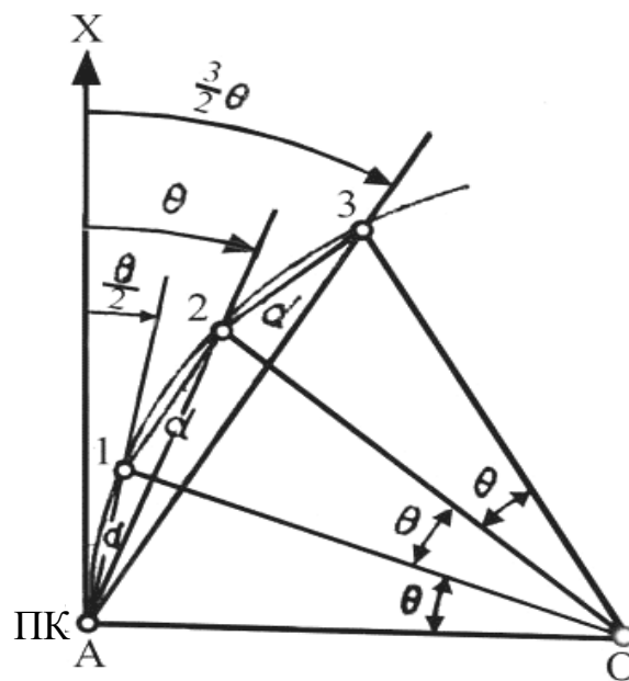
Рис. 6.4. Спосіб полярних координат
