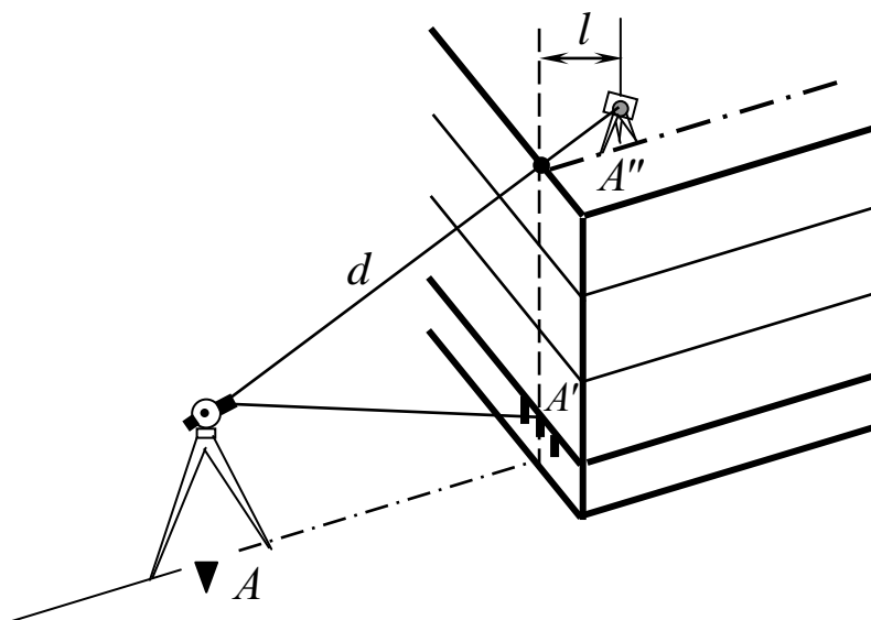
Рис. 8.22. Спосіб похилого проектування
