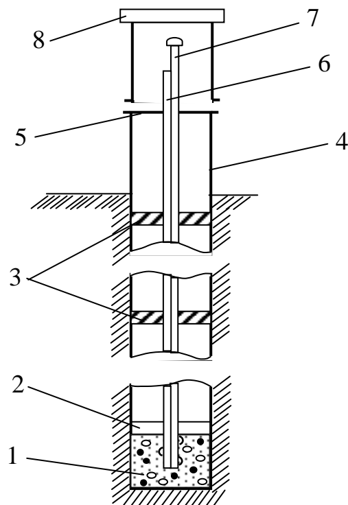
Рис. 9.1. Біметалічний глибинний репер
