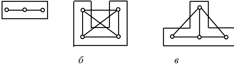
Рис. 4.1. Найпростіші базисні фігури внутрішньої геодезичної розмічувальної мережі
