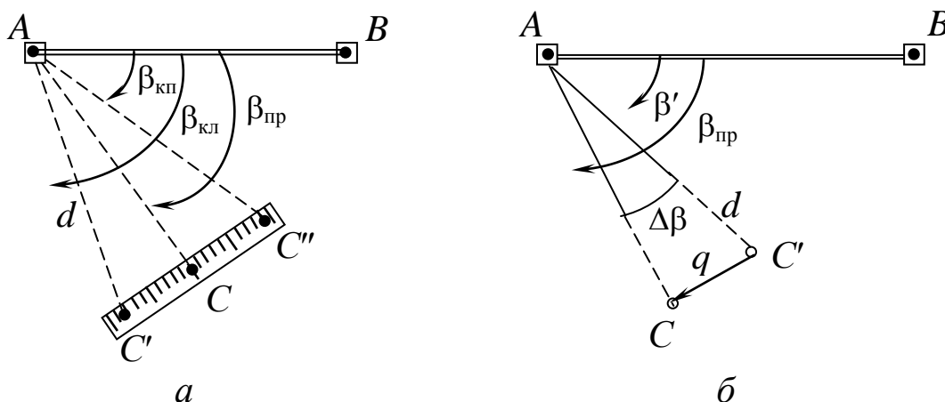
Рис. 5.1. Побудова проектного кута
