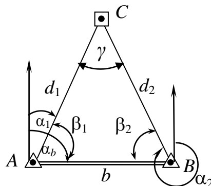
Рис. 2.12. Одноразова лінійна засічка
