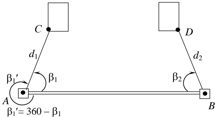
Рис. 5.4. Спосіб полярних координат
