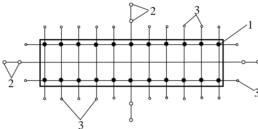
Рис. 8.5. Схема закріплення головних та допоміжних осей промислового будинку:
