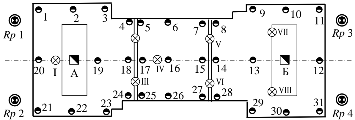
Рис. 9.3. Проект розміщення контрольних марок
