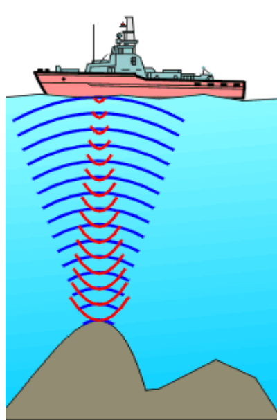
Рис. 3.16. Принцип знімання ехолотом
