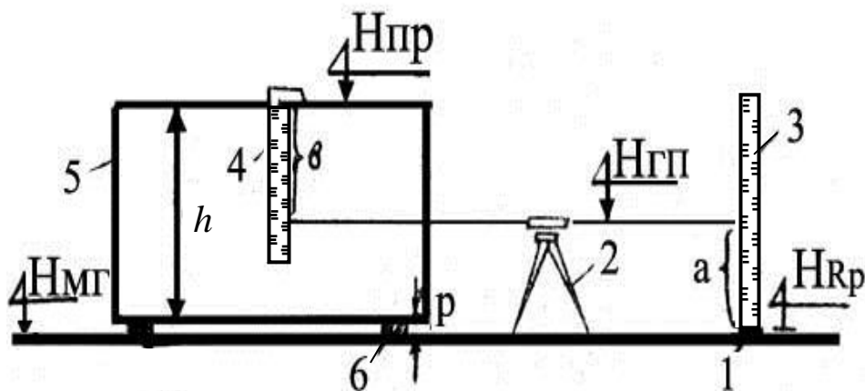
Рис. 7.9. Схема монтажу й вивірки панелі по висоті
