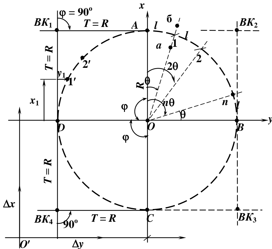
Рис. 6.7. Розмічування кола
