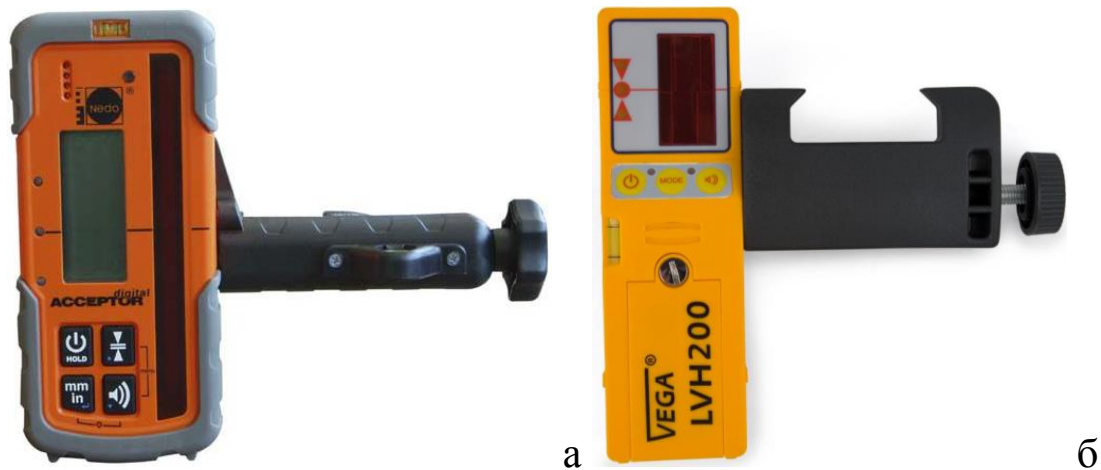
Рис. 1.19. Приймачі лазерного випромінювання
