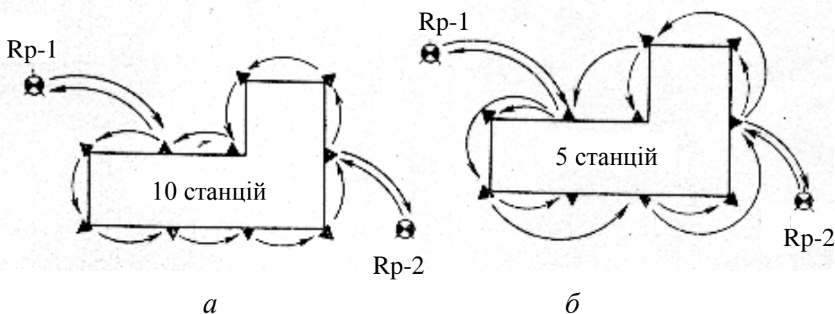
Рис. 9.4. Схема нівелювання осадочних марок
