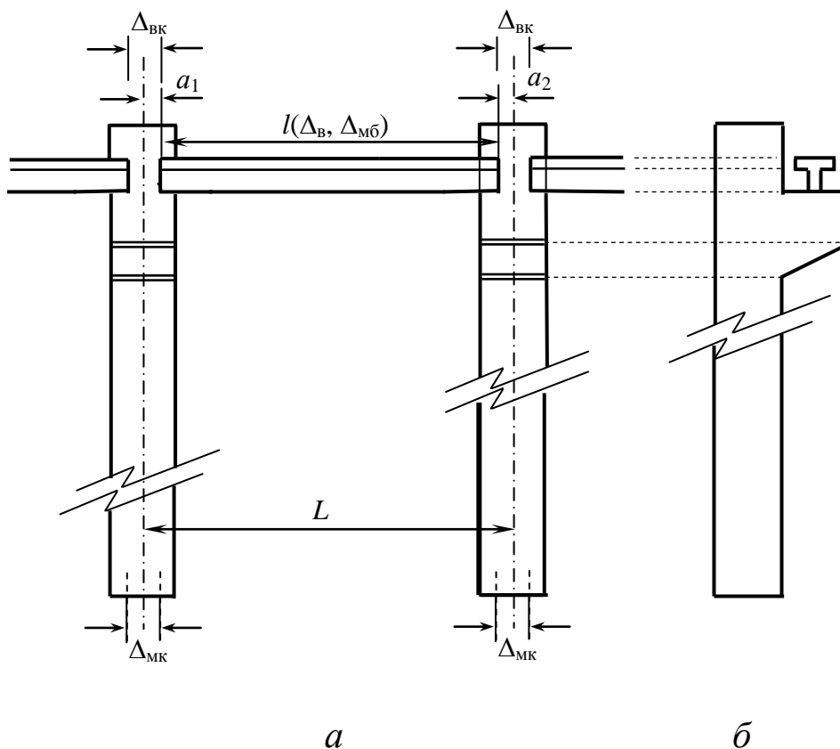
Рис. 4.14. Схема сполучення елементів конструкції а – повздовжній переріз; б – поперечний переріз
