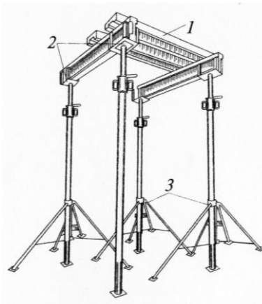
Рис. 8.29. Схема зведення монолітного залізобетонного каркасу:
