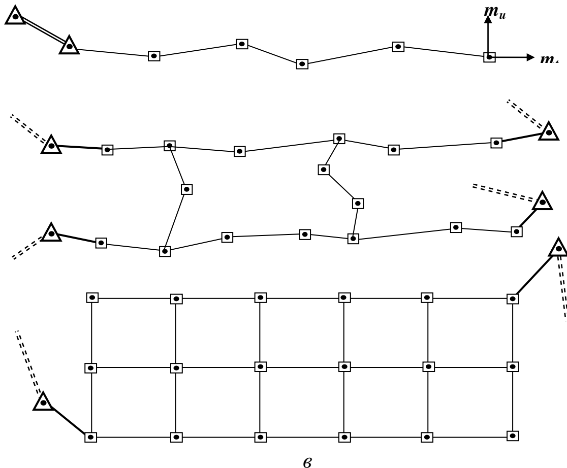
Рис. 2.7. Схеми мереж інженерної полігонометрії
