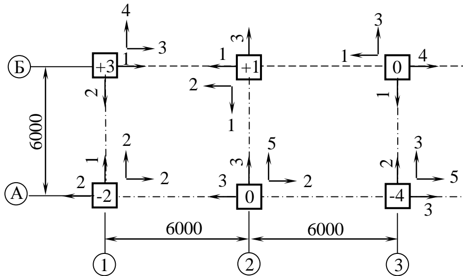
Рис. 8.53. Виконавча схема КОЛОН на монтажному горизонті
