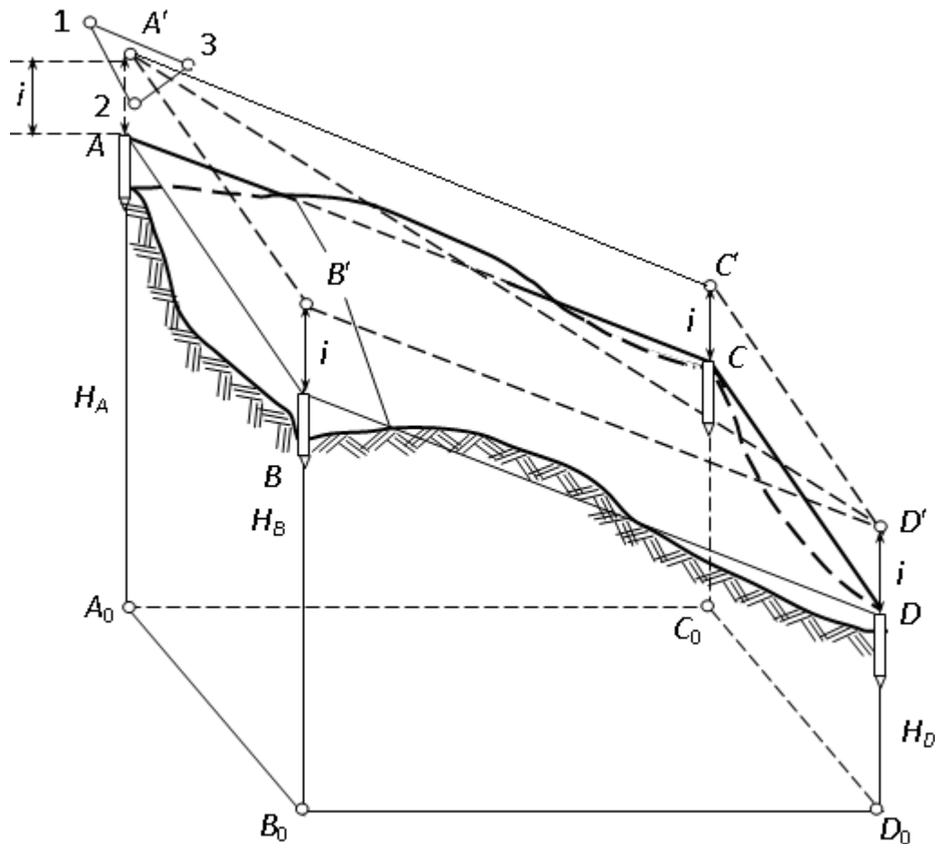
Рис. 5.14. Розмічування площини заданого нахилу
