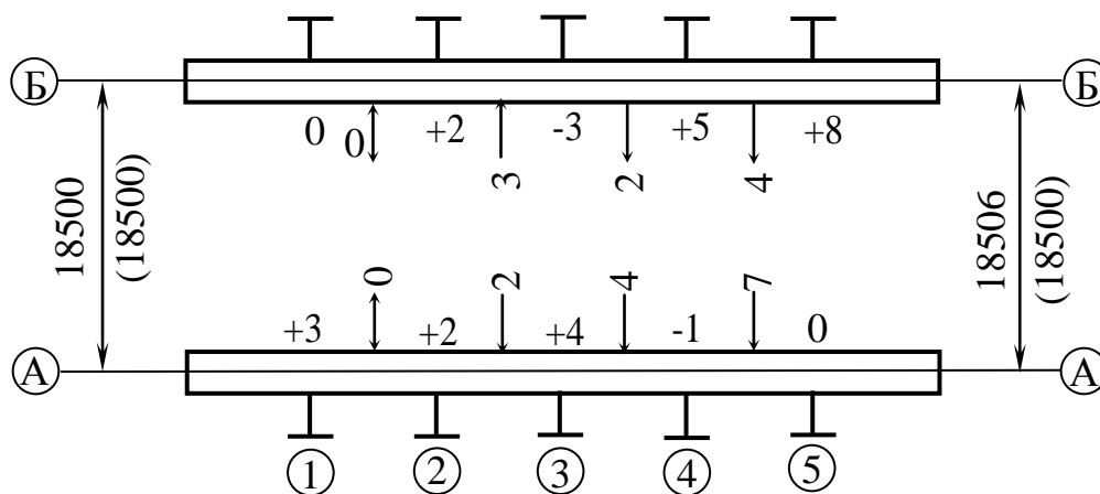
Рис. 8.54. Виконавча схема підкранових рейок мостового крану
