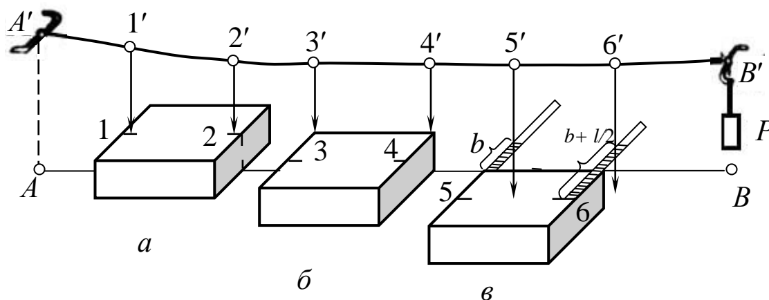
Рис . 7.7. Схема монтажу блоків в струнному способі:
