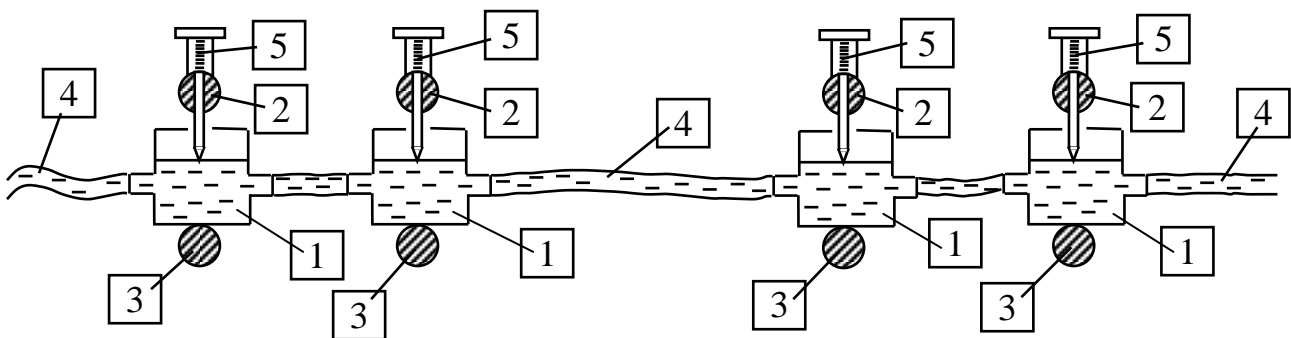
Рис. 9.5. Стаціонарна гідростатична система
