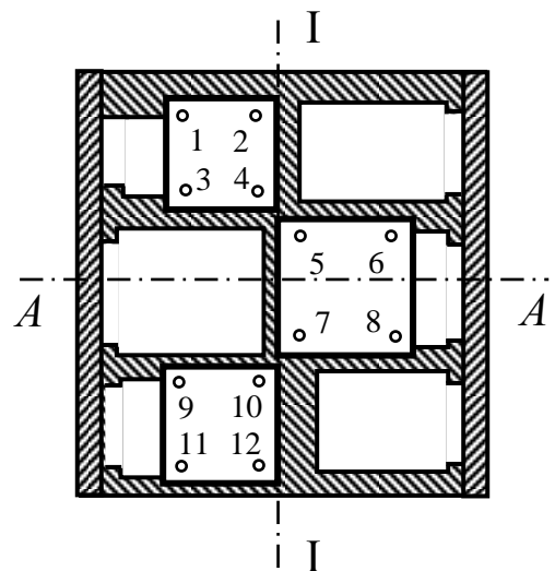
Рис. 8.19. Кондуктор
