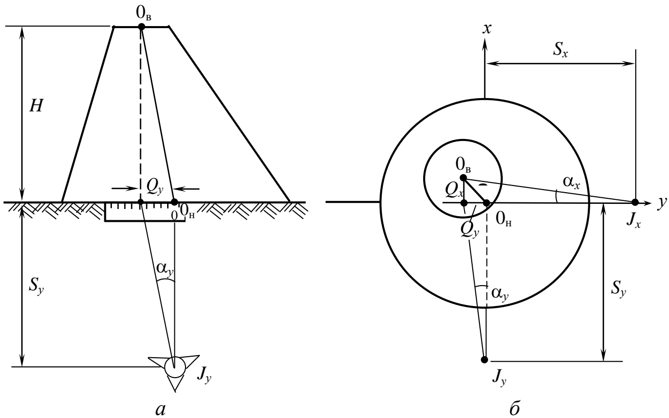
Рис. 9.10. Метод нахилого проектування
