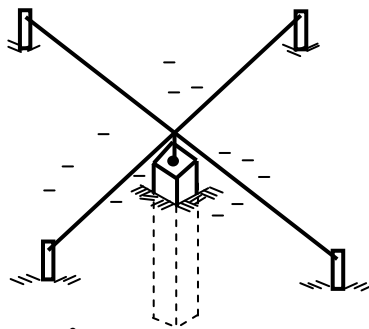
Рис. 4.9. Схема закріплення пункту будівельної сітки постійним знаком
