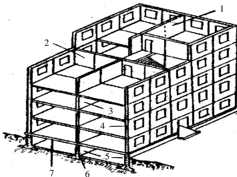
Рис. 8.25. Схема безкаркасного великопанельного будинку:
