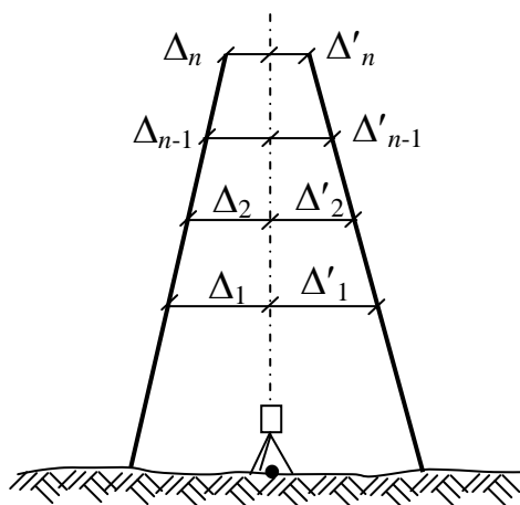
Рис. 9.8. Визначення крену баштової споруди методом вертикального проектування
