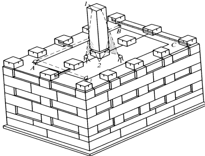
Рис.8.30. Схема геодезичних розмічувальних робіт на монтажному горизонті
