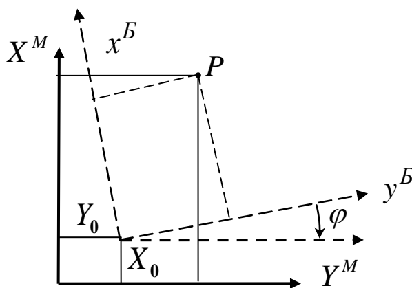
Рис. 2.1. Перетворення між місцевою та будівельною системами координат
