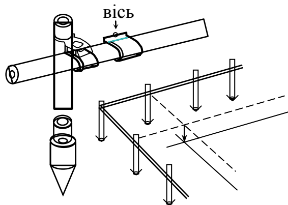
Рис. 8.9. Інвентарна обноска
