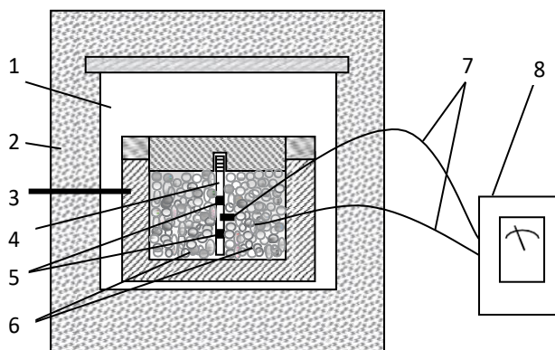
Рис. 1. Схема експериментальної установки для визначення теплофізичних характеристик зерна: 1 – термокамера; 2 – теплоізоляційний матеріал; 3 – вимірювальна камера, 4 – латунна пластина (зонд); 5 – ебонітова рамка; 6 – насіння; 7 – термомпари; 8 – потенціометр.
