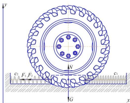
Рис. 2. Динамічна модель кочення колісного рушія.
