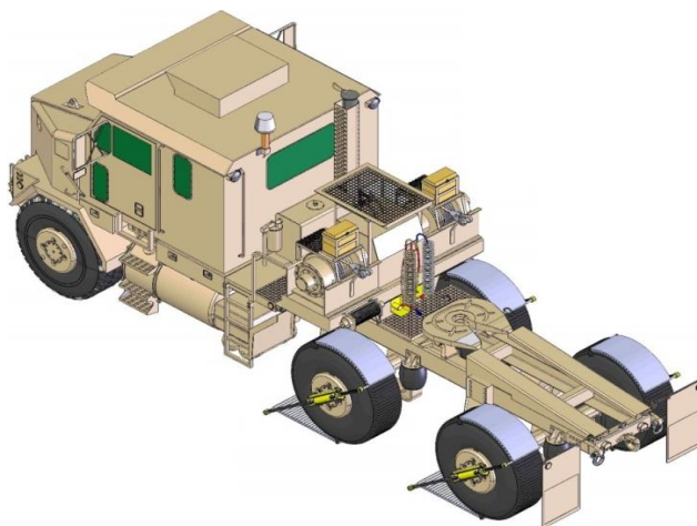
Рис.3. Загальний вигляд мобільного енергетичного засобу з конструктивним вдосконаленням колісного рушія.
