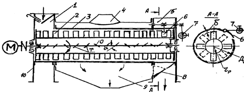
Рис.1. Принципова схема машини: 1 - живильник; 2 - лопатка; 3 - сито; 4 - патрубок аспірації; 5 - вихідний патрубок; 6 - клапан; 7 - противага; 8 - клапан перекидний; 9 - збірник; 10 – станина.
