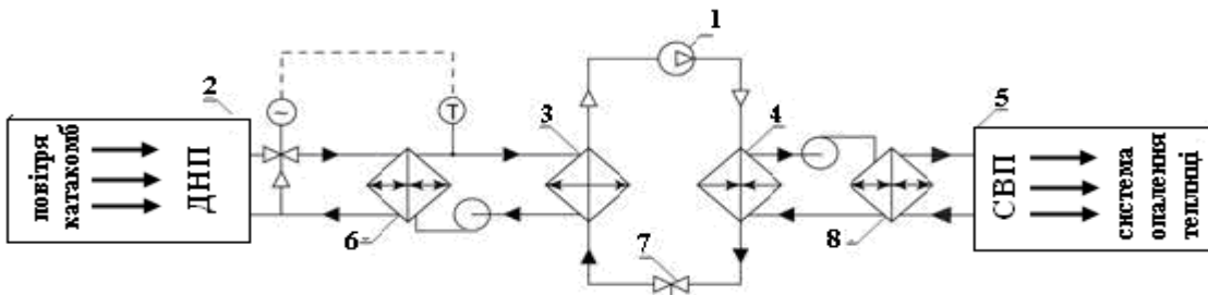
Рис. 2. Схема теплонасосної установки: 1- компресор; 2- джерело теплоти нижчого потенціалу (ДНП); 3- випарник теплового насоса; 4- конденсатор теплового насоса; 5- споживач теплоти високого потенціалу (СВП); 6- низькотемпературний теплообмінник; 7- регулятор потоку холодоагенту; 8- високотемпературний теплообмінник.
