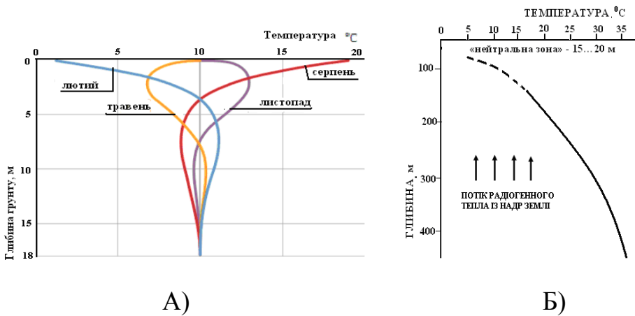
Рис. 1. Коливання температури ґрунту по глибині. А – в нейтральній зоні; Б – нижче нейтральної зони.
